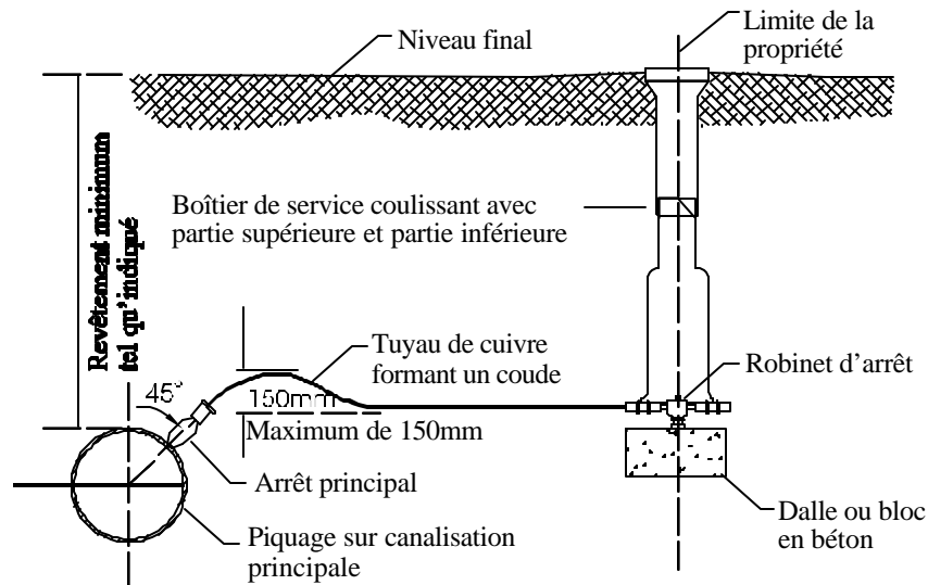
Figure 7 : Branchement d'alimentation en eau.
