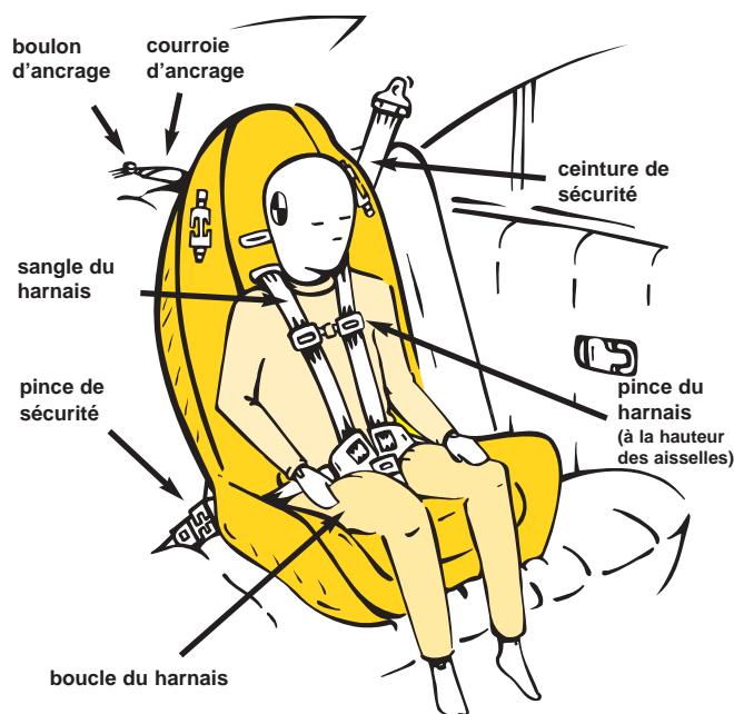
Siège d'enfant/siège d'appoint utilisé comme un siège d'enfant orienté vers l'avant
