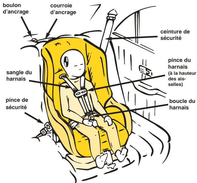
Siège d'enfant/de bébé utilisé face à l'avant
