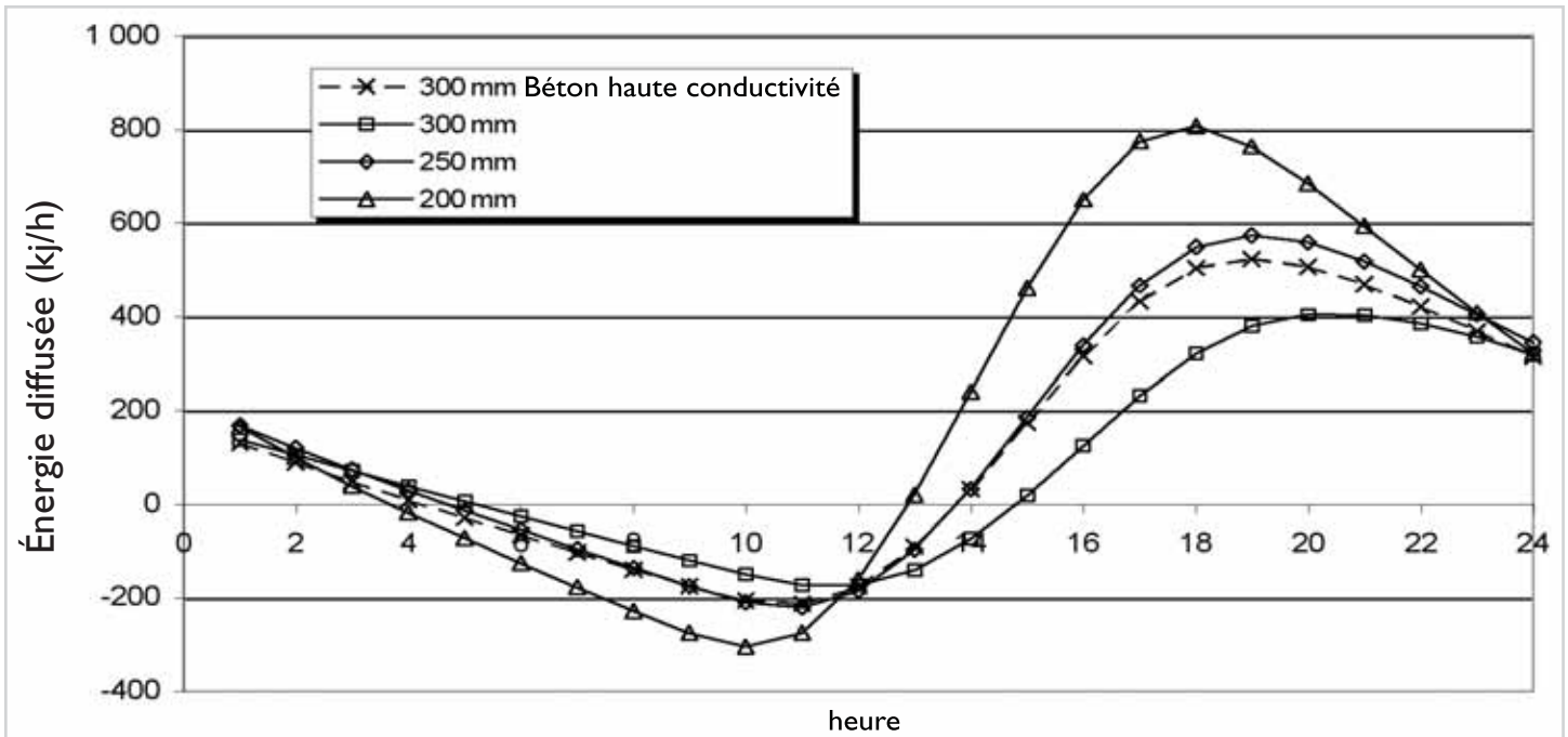
Figure 5 Énergie diffusée (kJ/h) vers l'intérieur d'une maison à Vancouver pendant une journée d'hiver par temps dégagé
