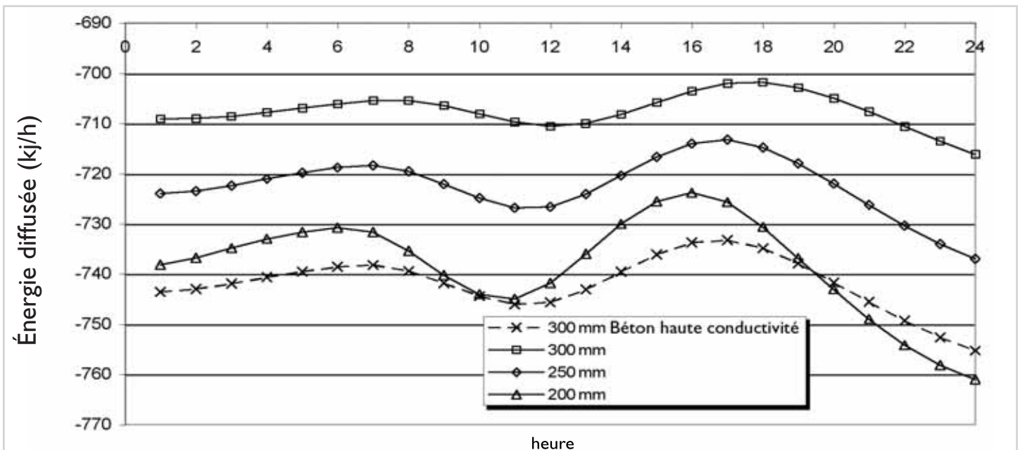
Figure 6 Énergie diffusée (kJ/h) vers l'intérieur d'une maison à Vancouver lors d'une journée typique d'hiver par temps nuageux
