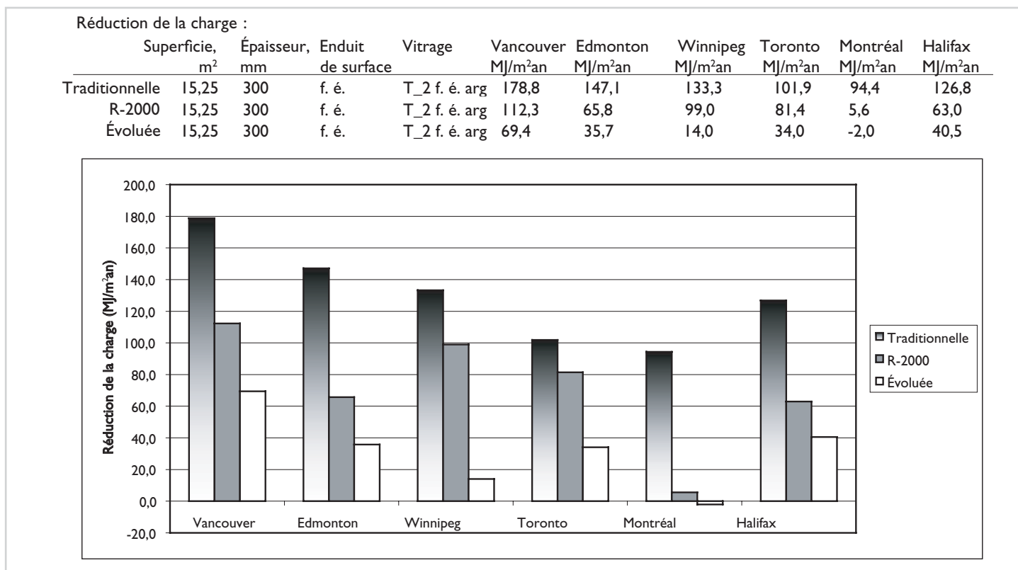
Figure 3 Réduction de la charge de chauffage pour les trois archétypes, par emplacement
