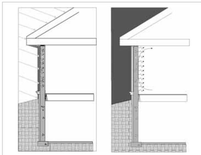
Figure 1 Mur de masse le jour et la nuit
