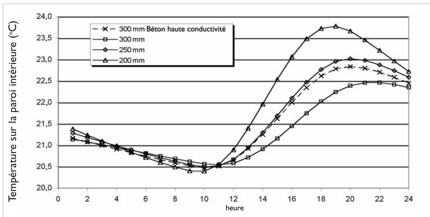
Figure 4 Échantillon des températures de la paroi intérieure (celsius) d'une maison R-2000 dans la région de Vancouver lors d'une journée de printemps
