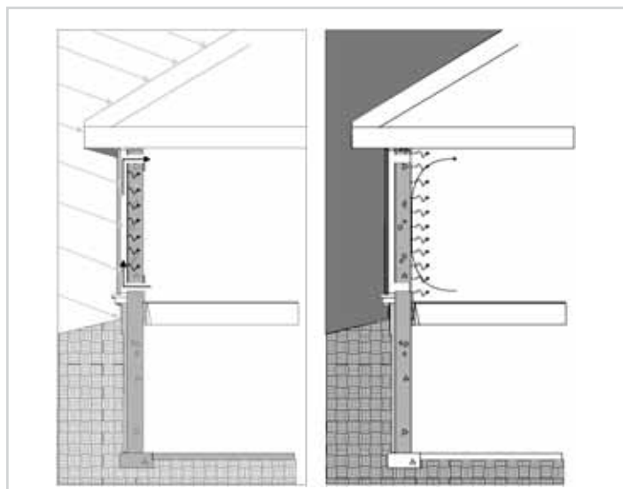
Figure 2 Mur Trombe le jour et la nuit
