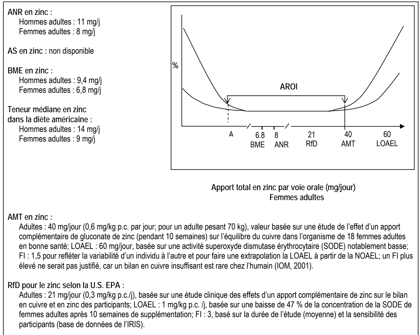
Figure 2 Comparaison de l'apport maximal tolérable (AMT) et de la dose de référence (RfD) pour le zinc
