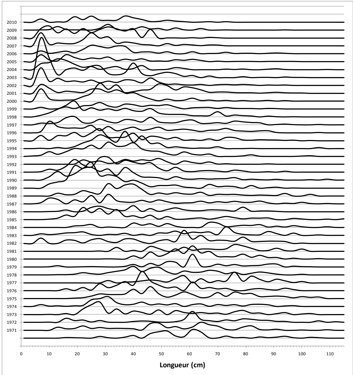
Figure 19. Fréquence des longueurs des loups atlantiques sur le plateau néo-écossais, établie d'après les données du relevé scientifique estival au chalut des Maritimes (estimations de l'abondance totale fondées sur un échantillonnage aléatoire stratifié). Voir le texte pour les biais liés aux changements d'engin.
