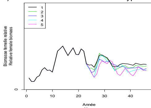
D) Sous-estimation de l'erreur d'observation
