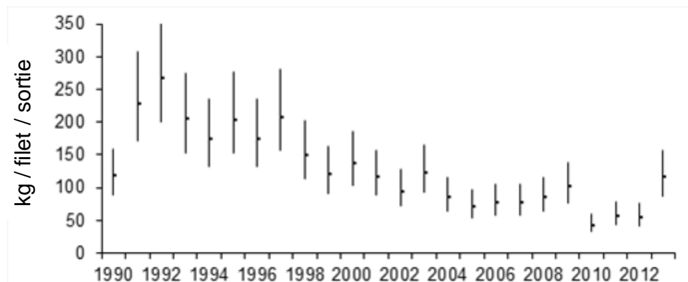
Figure 10. Indice des PUE pour les reproducteurs de printemps de 1990 à 2013 (kg / filet / sortie; moyenne et barres de plus ou moins deux erreurs-types).
