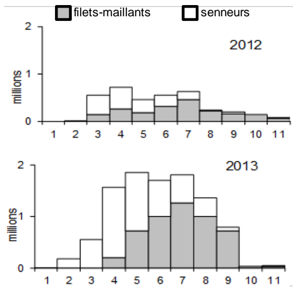
Figure 3. Prises selon l'âge des reproducteurs de printemps (millions de harengs) pour 2012 et 2013.
