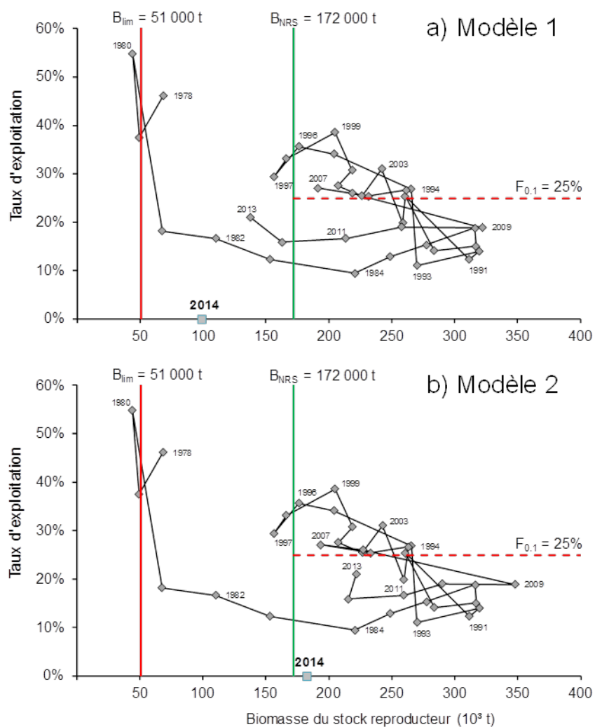
Figure 20. Biomasse du stock des reproducteurs d'automne (âges 4 +, t) et trajectoires du taux d'exploitation (% , âges 5 à 10) par rapport aux niveaux de référence selon : a) le modèle 1 (en haut), b) le modèle 2 (en bas). La biomasse du stock reproducteur pour 2014 est représentée par le symbole placé sur l'axe des abscisses.
