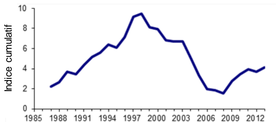
Figure 5. Indice cumulatif de l'abondance des reproducteurs de printemps, de 1987 à 2013, tiré du sondage téléphonique.
