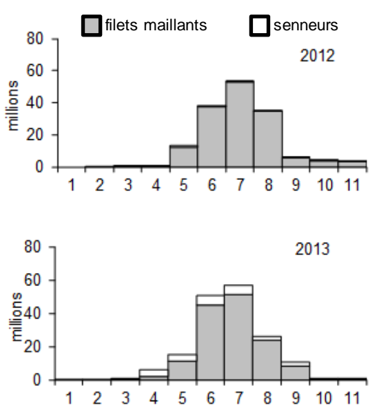
Figure 7. Prises selon l'âge des reproducteurs d'automne (millions de harengs) pour 2012 et 2013.
