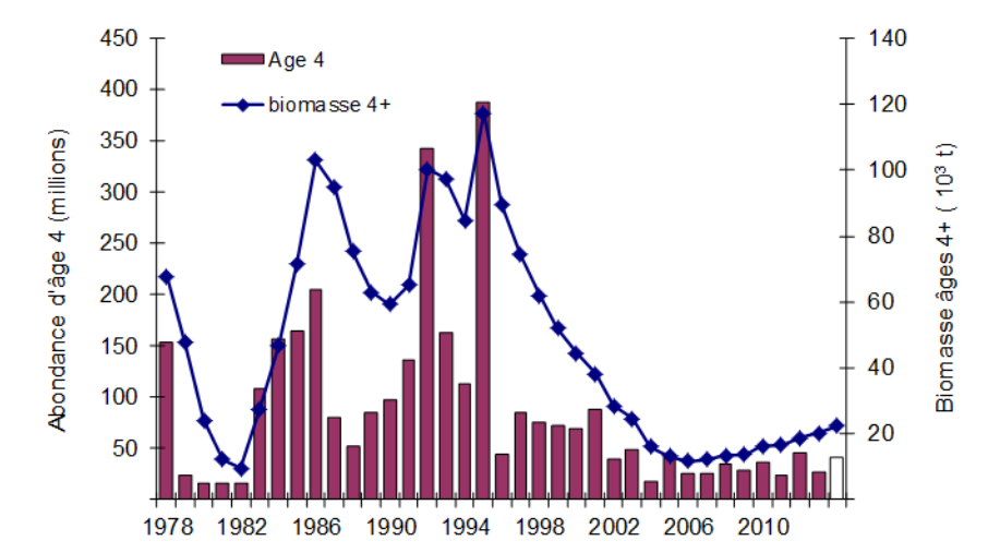
Figure 12. Nombre d'individus d'âge 4 de la composante des reproducteurs de printemps (millions de harengs) et biomasse du stock reproducteur des âges 4+ (en 10^3 t) au début de l'année, de 1978 à 2014. La valeur de l'abondance à l'âge 4 en 2014 est une estimation fondée sur le taux moyen de recrutement des cinq années précédentes.
