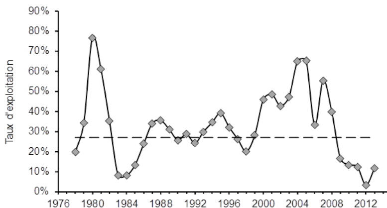
Figure 13. Taux d'exploitation des reproducteurs de printemps (en pourcentages, pour les âges 6 à 8) de 1978 à 2013. La ligne horizontale pointillée représente le taux d'exploitation de référence de 27 % correspondant à F_{0,1} .
