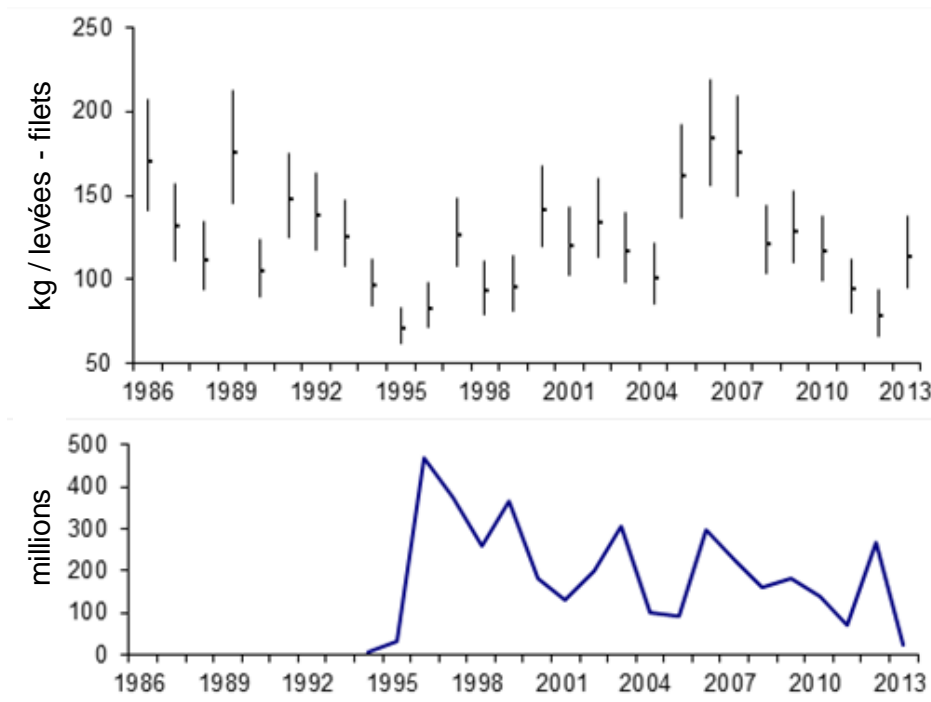
Figure 17. Indice du taux de prise (PUE ;kg/ levées-filets) des reproducteurs d'automne de 1986 à 2013 (graphique du haut) et indice (millions) du relevé acoustique pour les âges 2 et 3 de 1994 à 2013 (graphique du bas).
