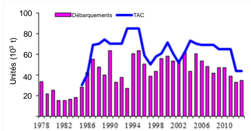
Figure 6. Total des débarquements (t) et total autorisé des captures (TAC; t) de la composante des reproducteurs d'automne du hareng de l'Atlantique de la division 4T de l'OPANO, de 1978 à 2013.
