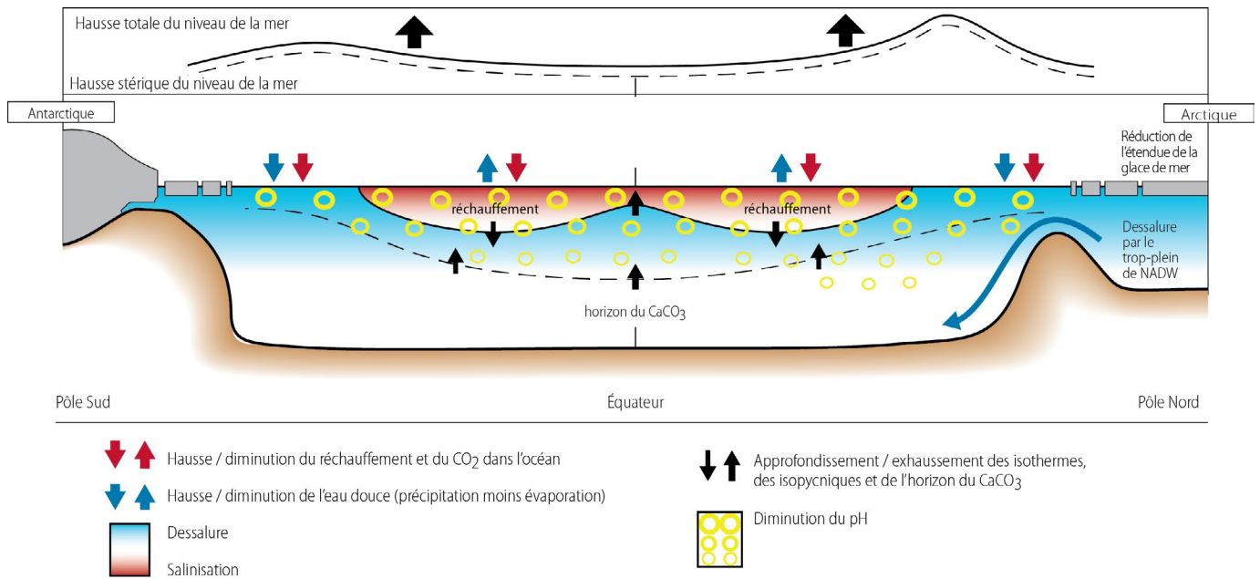
FIGURE 24 : Profil schématique des principaux changements climatiques observés dans l'océan. La légende indique s'il s'agit d'une hausse ou d'une baisse. Dans le texte, l'élévation du niveau « total » de la mer fait référence à l'élévation du niveau « absolu » de la mer, et l'« horizon » du CaCO 3 (carbonate de calcium), à la « profondeur de saturation » (source : Bindoff et al. , 2007).
