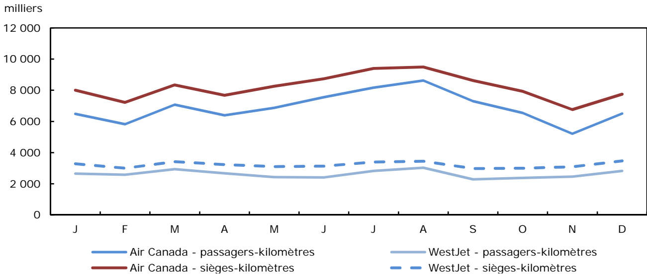
Graphique 2 Passagers-kilomètres et sièges-kilomètres, services réguliers, Air Canada et WestJet, janvier à décembre 2013
