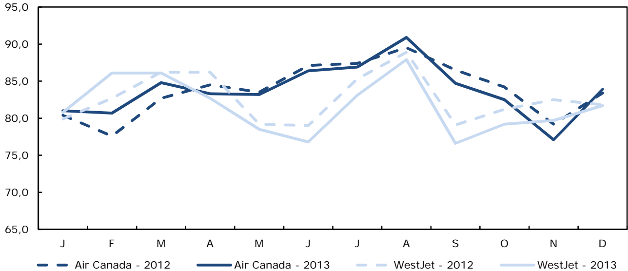
Graphique 6 Heures de vol et consommation de carburant à turbomoteurs, Air Canada et WestJet, janvier à décembre 2013
