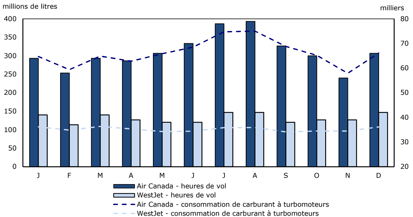
Graphique 6 Heures de vol et consommation de carburant à turbomoteurs, Air Canada et WestJet, janvier à décembre 2014
