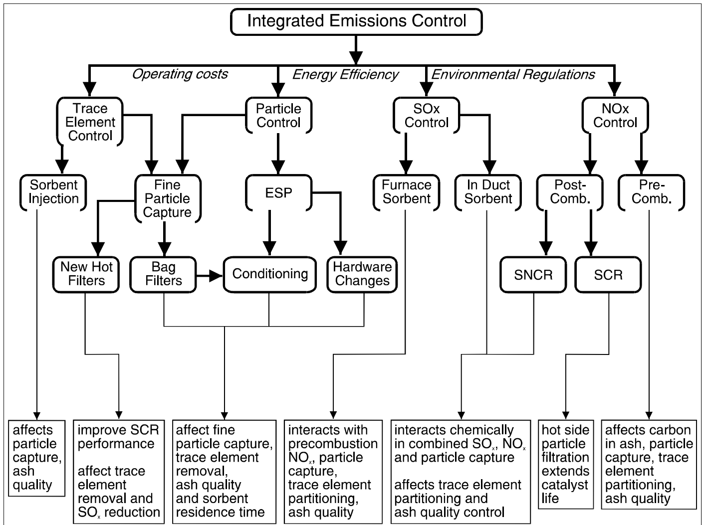
Procédés interactifs de réduction des polluants atmosphériques provenant de la combustion de combustibles
