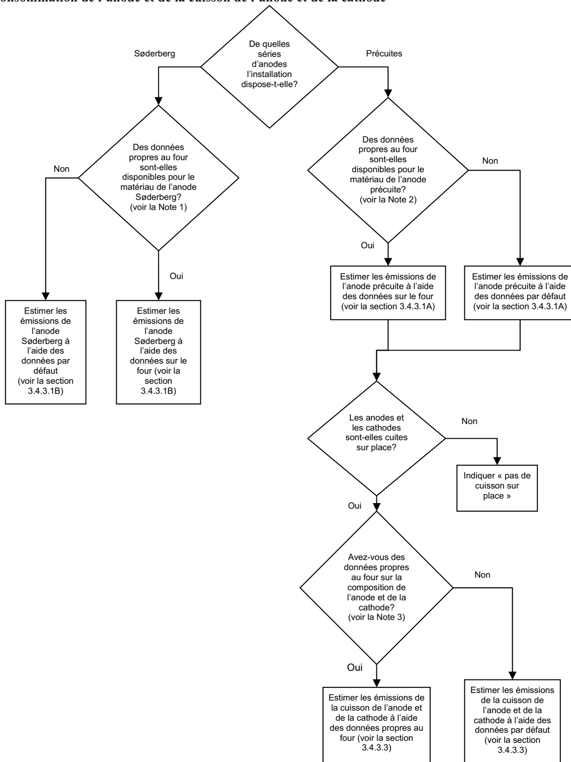
Figure 3 : Organigramme pour choisir la méthode d'estimation des émissions de CO 2 provenant de la consommation de l'anode et de la cuisson de l'anode et de la cathode
