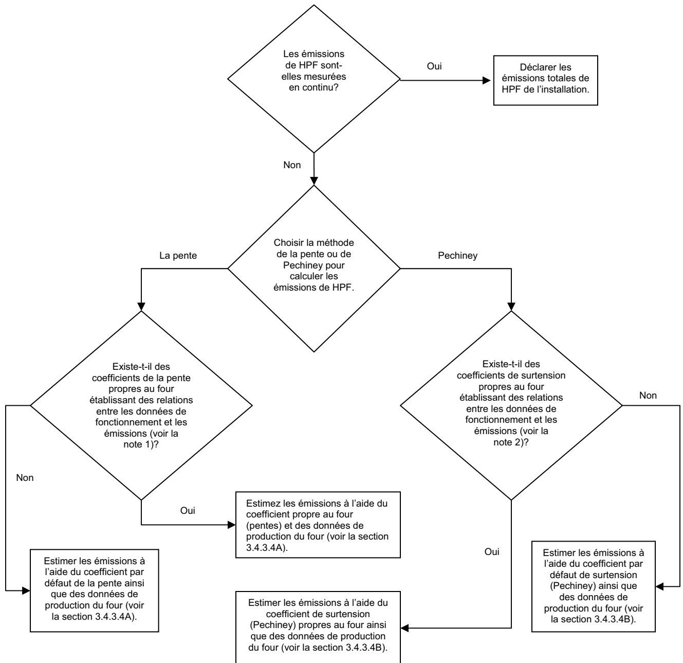
Figure 4 : Organigramme pour choisir la méthode d'estimation des émissions de HPF résultant des effets d'anode
