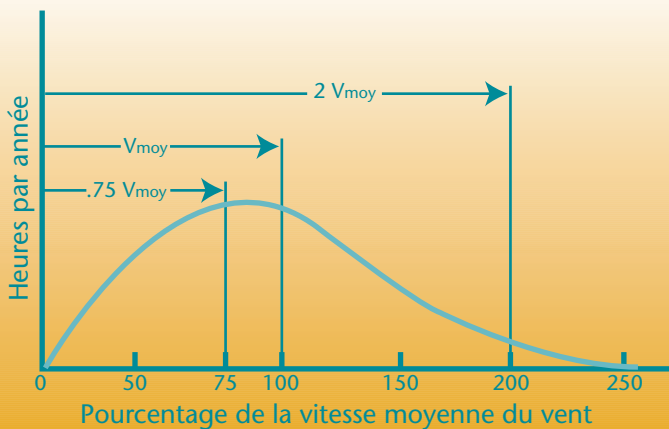
▲ Figure 3. Vitesse annuelle moyenne du vent ( V_{moy} ). Le point le plus élevé de la courbe correspond à la vitesse à laquelle le vent souffle la plus souvent. Ce type de graphique est appelé courbe Rayleigh de distribution de la vitesse du vent.
