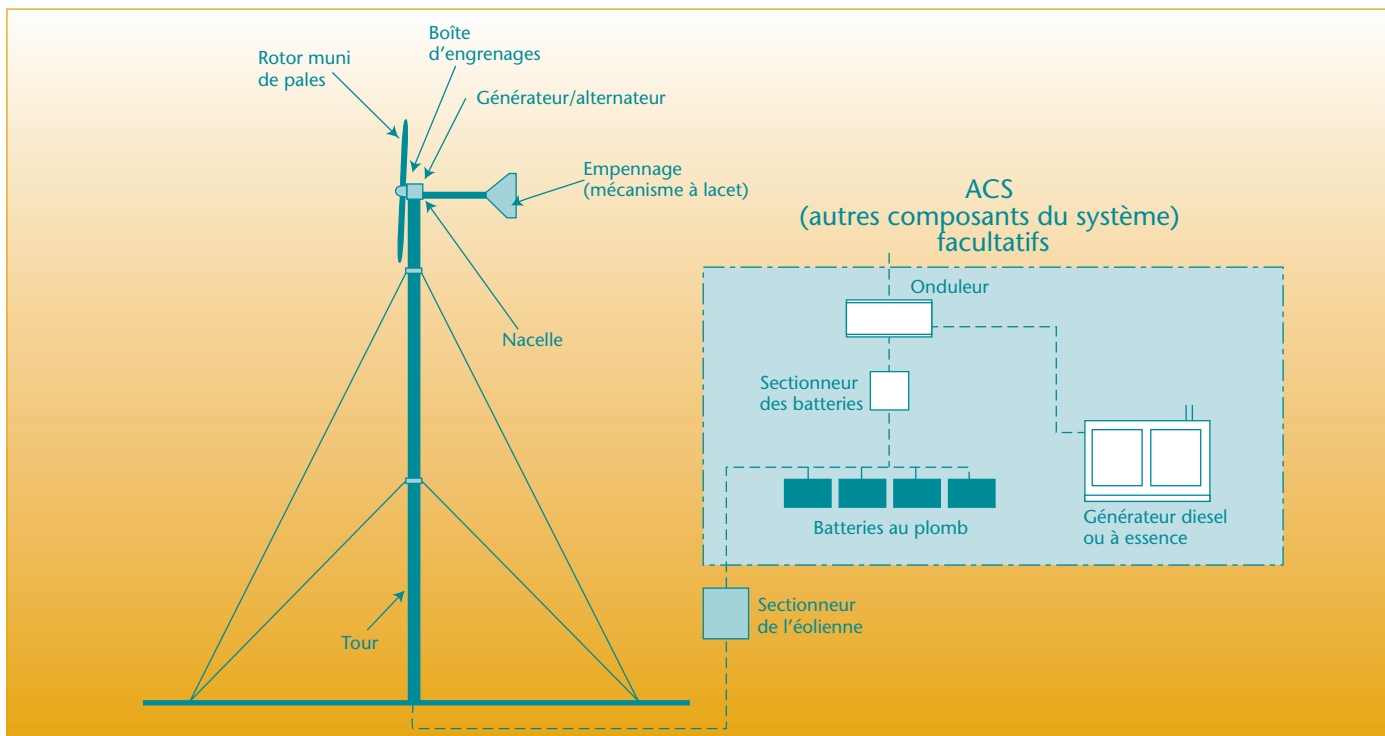
▲ Figure 6. Composants du système éolien.
