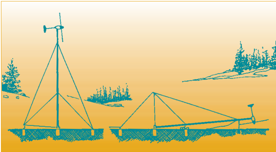
▲ Figure 7. Les tours basculantes s'abaissent jusqu'au niveau du sol, pour faciliter l'installation du générateur et son entretien.
