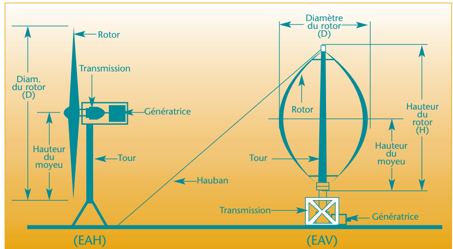
▲ Figure 5. Les éoliennes à axe horizontal (EAH) et à axe vertical (EAV).
