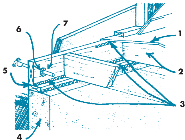
Détail de la lisse d'assise et de la solive de bordure
