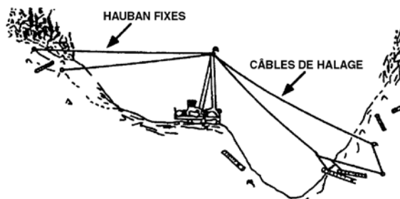
Figure 2.1 - Pylône articulé
