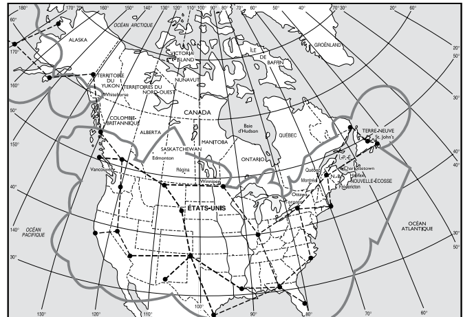
Figure 3.3 – Secteur de couverture estimé de LORAN-C pour un rapport signal/bruit 1:3
