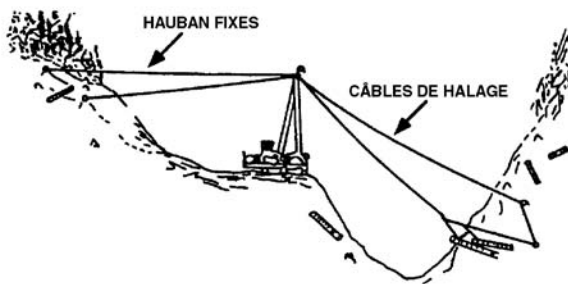
Figure 2.1 – Pylône articulé
