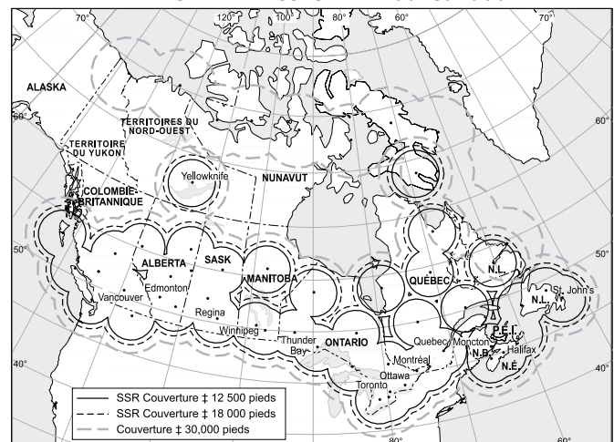
Figure 4.1 – Couverture radar fournie par NAV CANADA et le MDN au Canada
