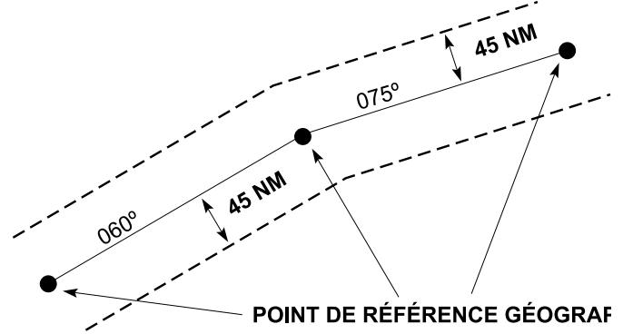
Figure 6.1 – Espace aérien à protéger le long des routes hors des voies aériennes
