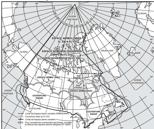
Figure 12.1 – Espace aérien CMNPS, espace aérien RNPIC et espace aérien de transition CMNPS
