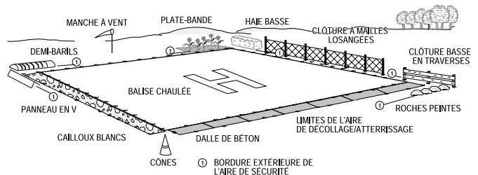
EXEMPLES DES DIFFÉRENTES BALISES D'UN HÉLIPORT GAZONNÉ
