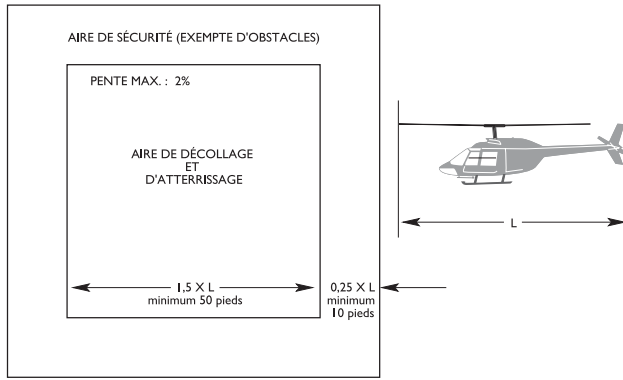
AIRE DE DÉCOLLAGE ET D'ATTERRISSAGE/AIRE DE SÉCURITÉ
