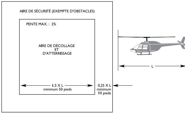
AIRE DE DÉCOLLAGE ET D'ATERRISSAGE/AIRE DE SÉCURITÉ
