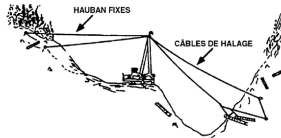
Figure 2.1 - Pylône articulé
