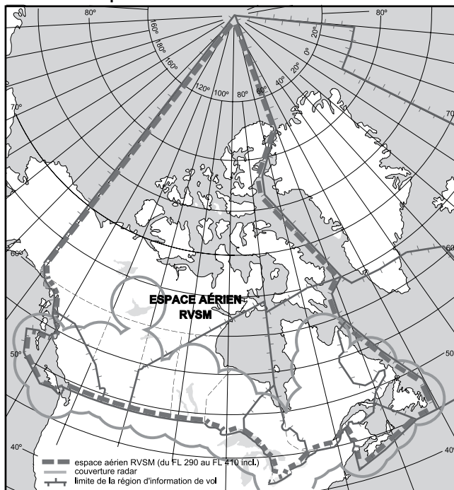
Figure 12.2 – Espace aérien RVSM et espace aérien de transition RVSM
