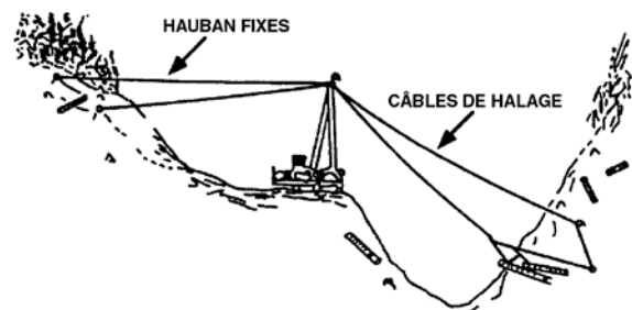
Figure 2.1 - Pylône articulé
