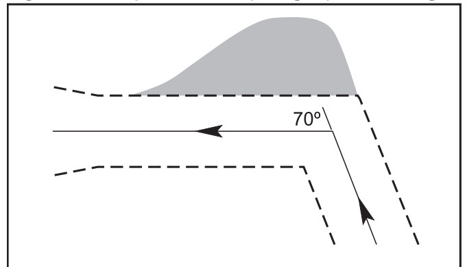
Figure 6.2 – Espace aérien à protéger pour les virages
