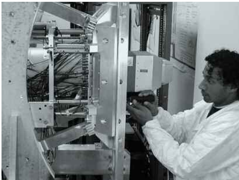
Installation du premier détecteur de rayons gamma du nouveau spectromètre TIGRESS, mis au point pour l'installation d'ions radioactifs accélérés ISAC-II.
