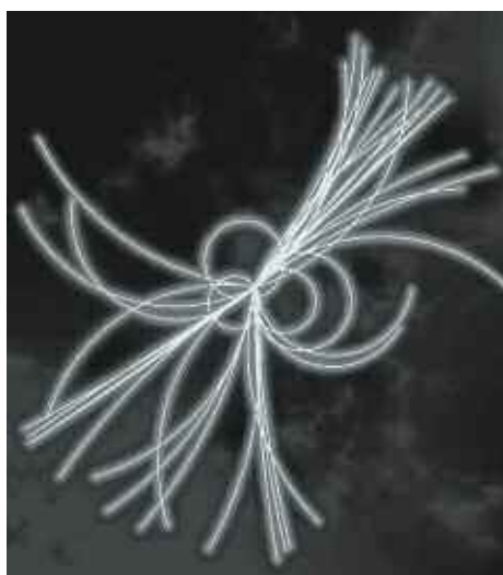
Simulation de particules émergeant de la désintégration d'une particule de Higgs, à la suite d'une interaction à haute énergie entre électrons et positrons.
