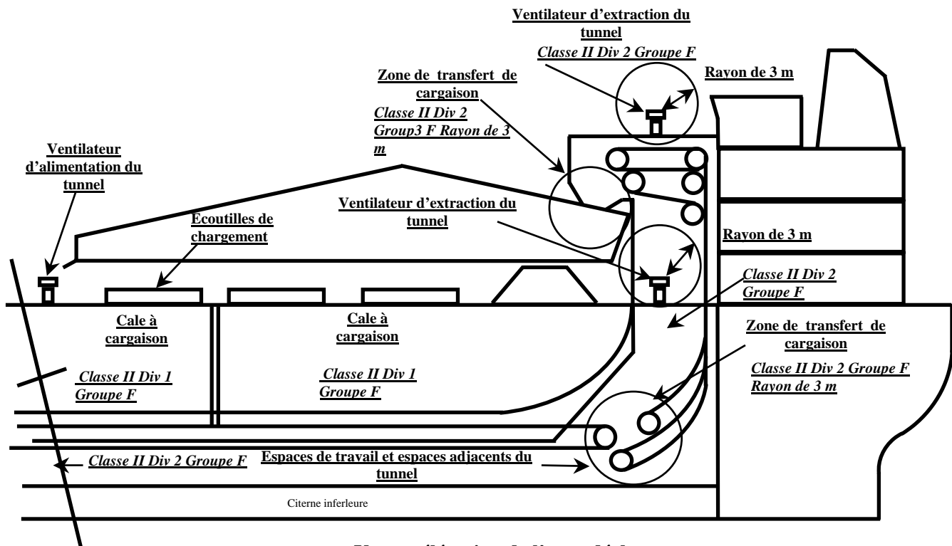
Vue en élévation de l'autodécharger
