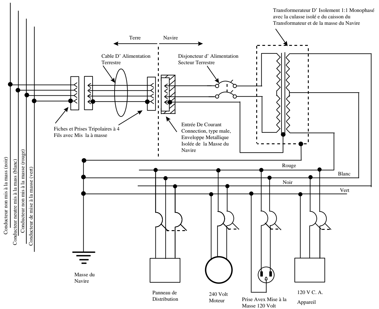
FIGURE 11-2 CIRCUIT D'UN TRANSFORMATEUR D'ISOLEMENT AVEC ENTRÉE MONOPHASE 240 VOLTS ET SORTIE MONOPHASÉE 120/240 VOLTS
