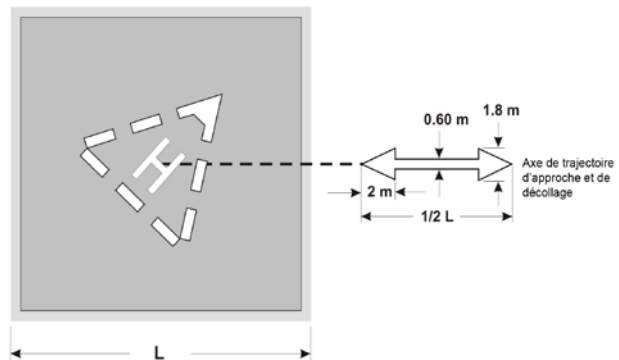
Marques de direction d'approche et de décollage
