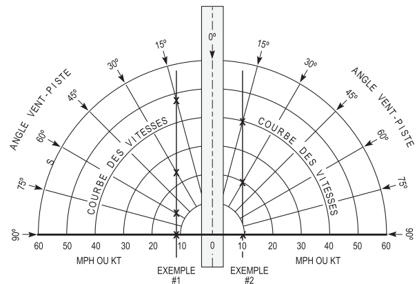
Exemple 1 : Aéronef ayant une vitesse de décrochage de 60 MPH VITESSES DE VENT
