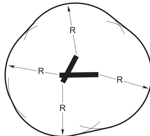
Figure 9.3 – Zone d'évolution à vue pour approche indirecte
