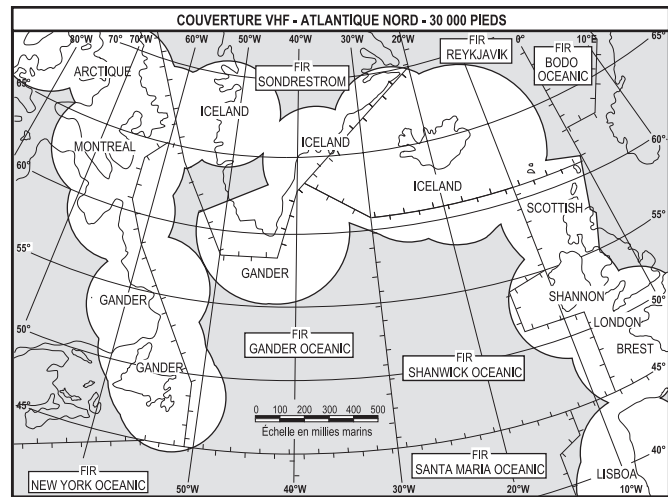
NOTE : L'altitude minimale pour une couverture VHF continue sur l'Atlantique Nord est de 30 000 pieds.
