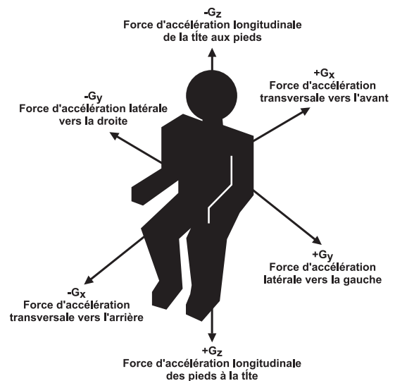
Figure 3.1 – Les axes de la force d'accélération
