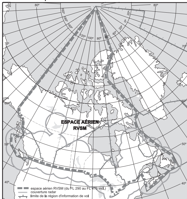
Figure 12.2 – Espace aérien RVSM et espace aérien de transition RVSM
