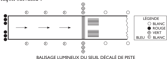
BALISAGE LUMINEUX DU SEUIL DÉCALÉ DE PISTE
