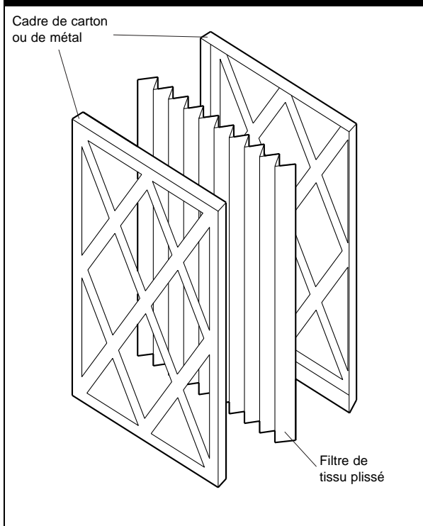
Figure 50 : Filtre plissé d'efficacité moyenne
