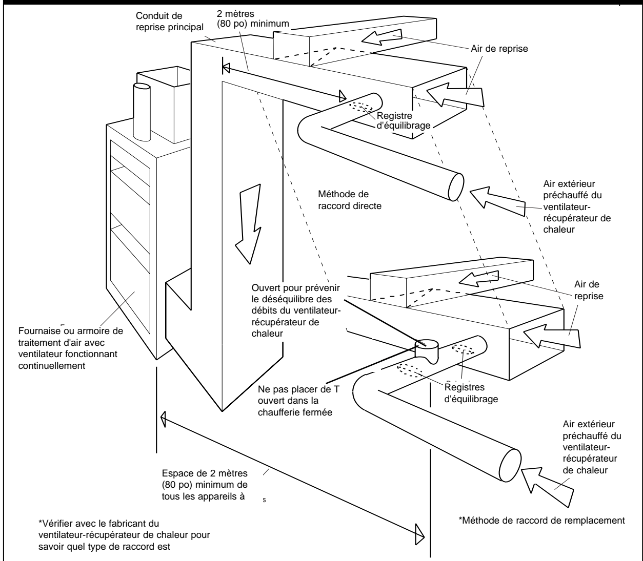
Figure 47 : Raccord RCV à système de chauffage à air pulsé
