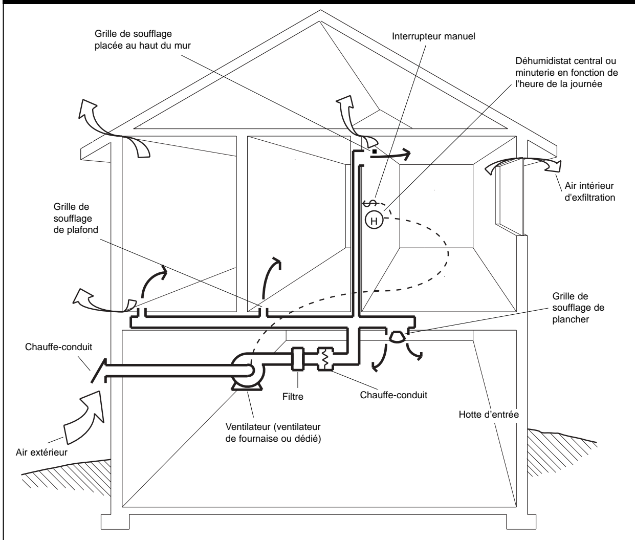
Figure 28 : Ventilation—Alimentation seulement
