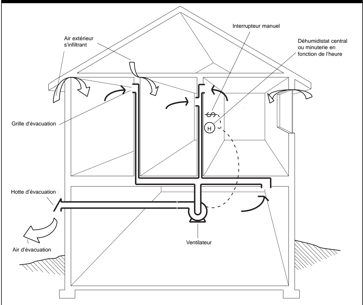
Figure 29 : Ventilation—Évacuation seulement
