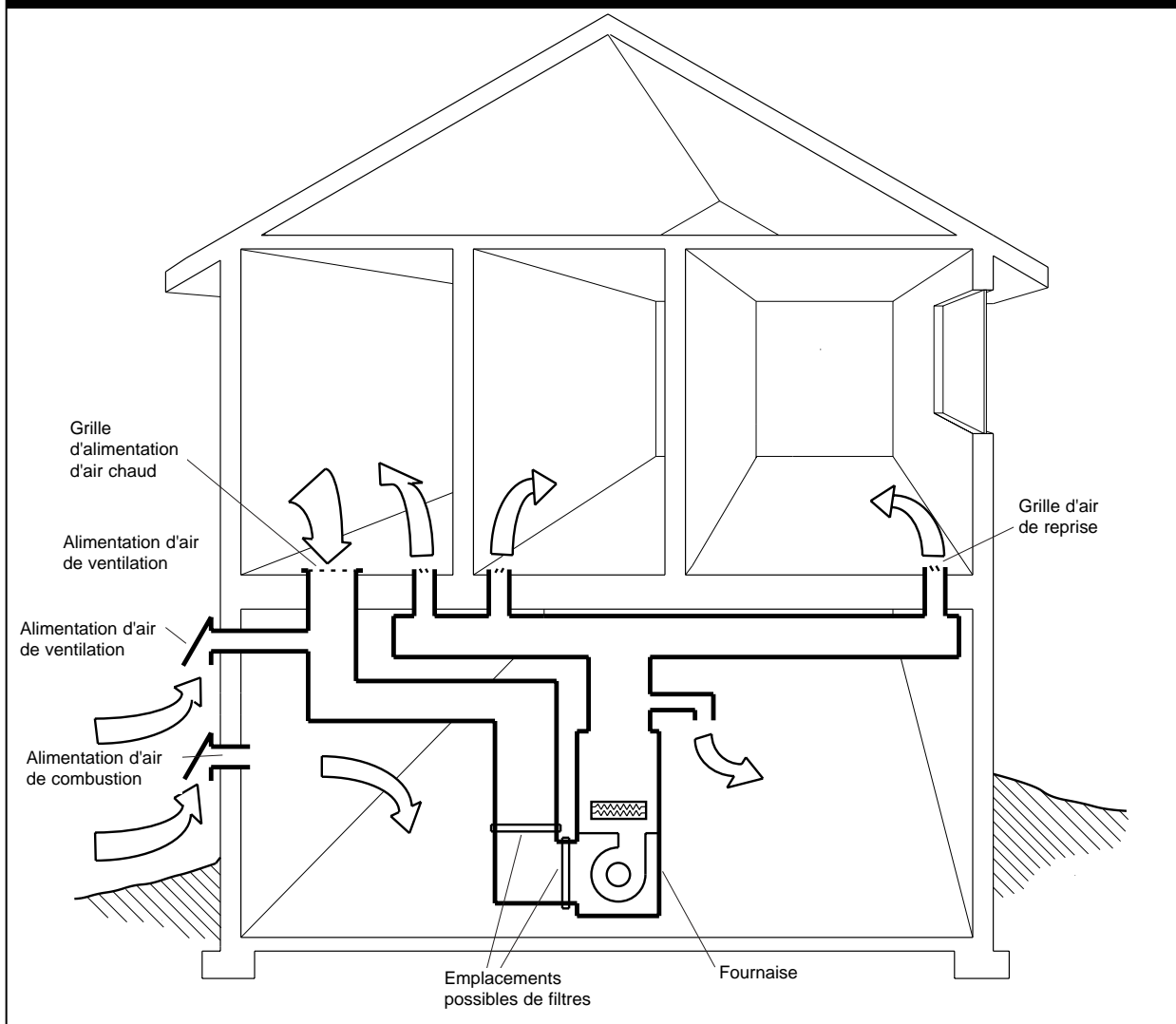
Figure 5 : Installation de chauffage à air chaud pulsé avec fournaise à aspiration naturelle
