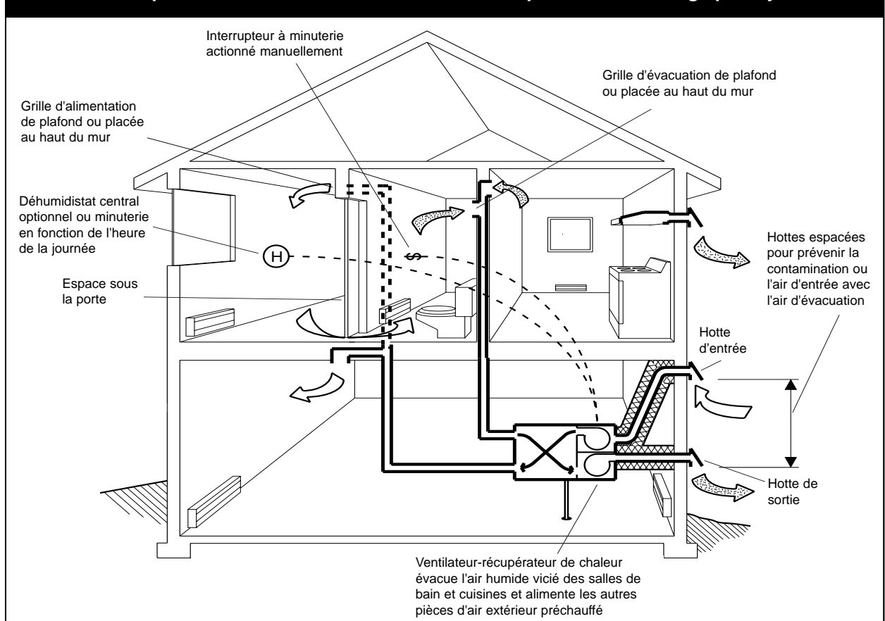
Figure 39 : Ventilateur-récupérateur de chaleur central à utiliser avec plinthe ou chauffage par rayonnement
