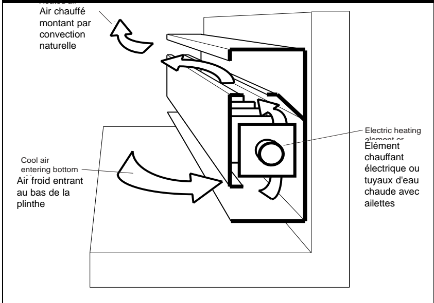
Figure 13 : Convecteur-plinthe
