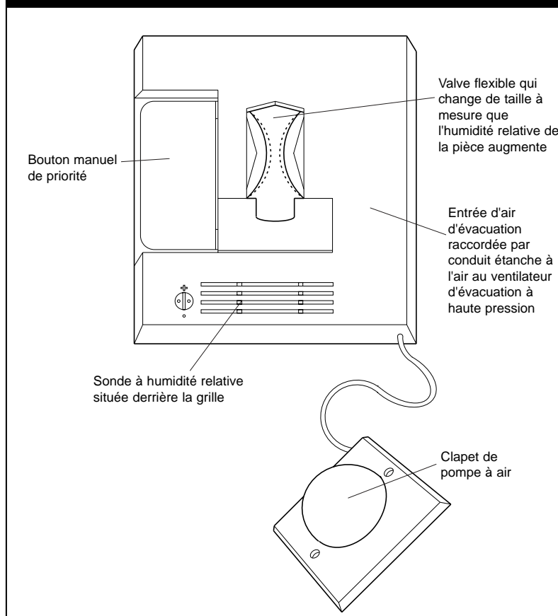
Figure 34 : Grille d'évacuation actionnée par l'humidité
