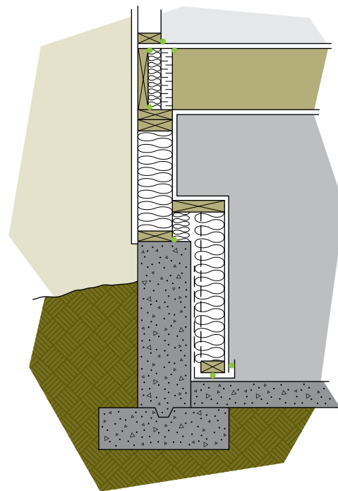
Figure 6-20 L'isolation d'un mur nain se fait en deux étapes et forme une pièce d'appui
