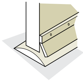
Coupe-bise à jupette
