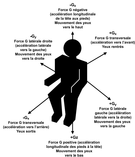
Figure 3.1 – Les axes de la force d'accélération
