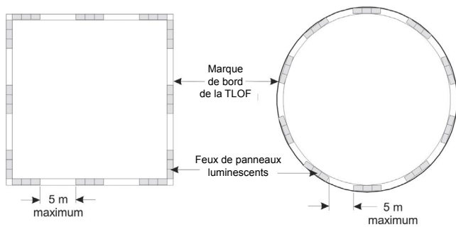
Exemples de balisage lumineux de la TLOF
