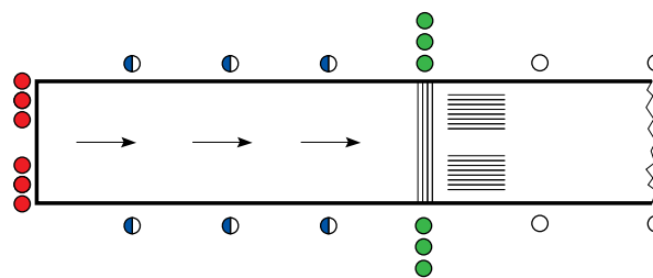
BALISAGE LUMINEUX DU SEUIL DÉCALÉ DE PISTE
