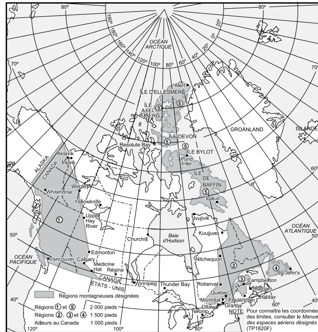
Figure 2.10 – Régions désignées montagneuses du Canada
