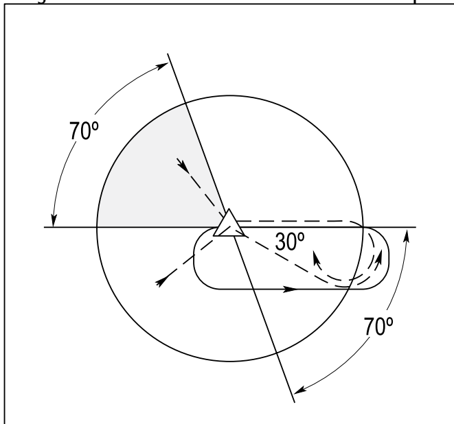
Figure 10.3 – Entrée dans un circuit non classique
