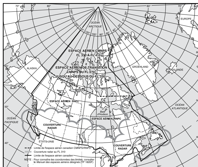
Figure 12.1 – Espace aérien CMNPS, espace aérien RNP et espace aérien de transition CMNPS
