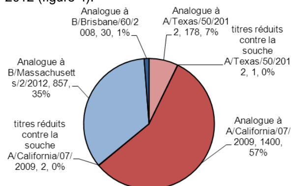
Figure 4. Caractérisation des souches grippales, Canada, 2013-14, N = 2 468
