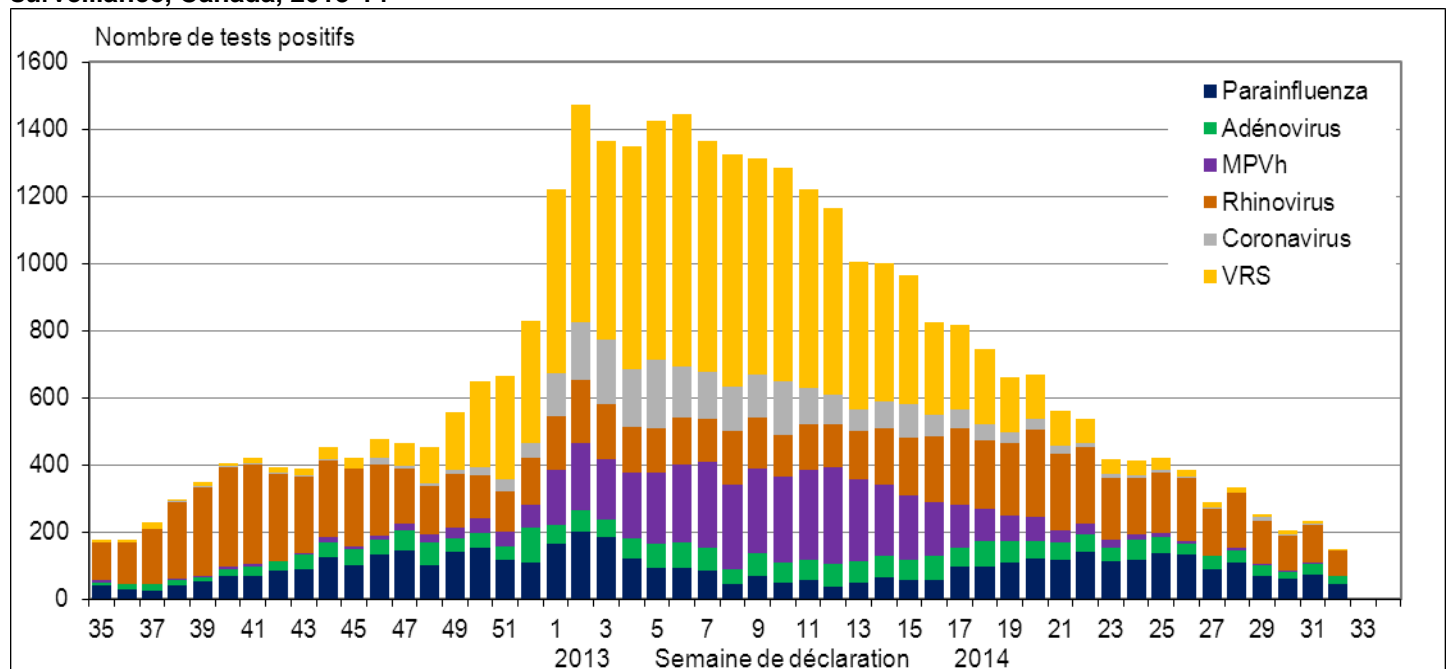
Figure 3. Nombre de tests de laboratoire positifs pour les autres virus respiratoires, par semaine de surveillance, Canada, 2013-14
