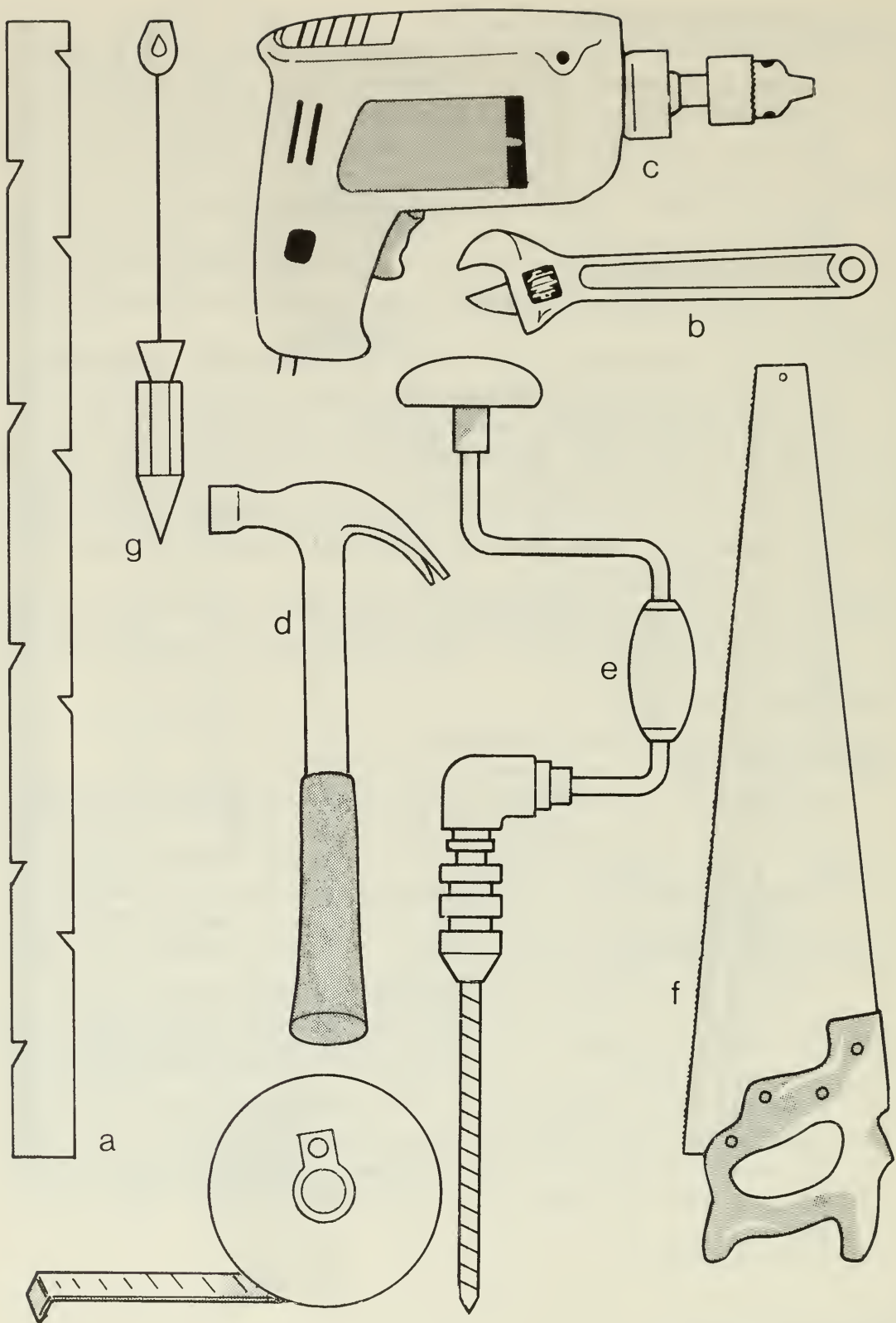
Fig. 14 Outils courants
