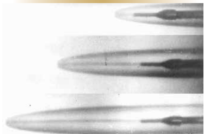
Figure 1 – Un projectile submergé qui se déplace à l'intérieur d'une supercavité autoformée a jusqu'à dix fois plus de vitesse qu'un projectile en contact direct avec l'eau de mer. (Y.N. Savchenko 2001)
