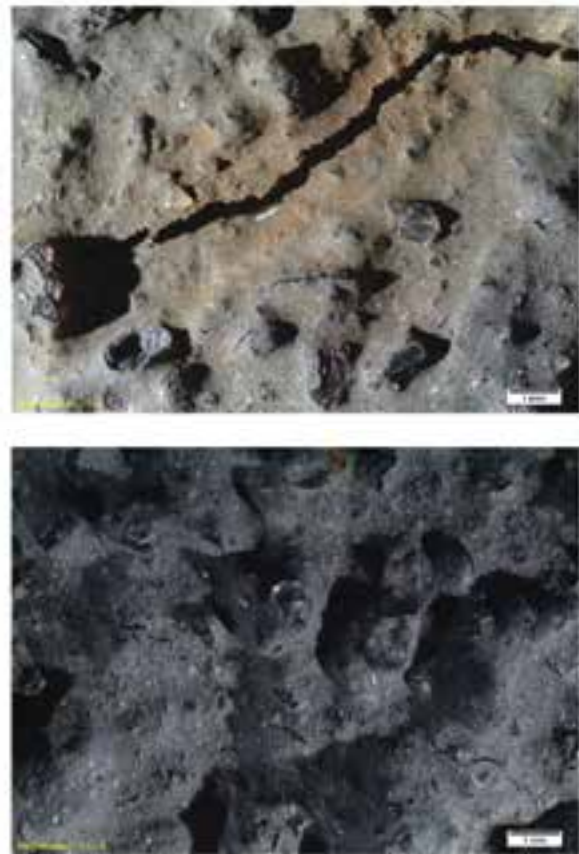
Figure 2 – Des images microscopiques de la surface du revêtement du pont. Les fissures correspondent à la détérioration d'un matériau qui a rétréci et subi des tensions internes. Aucun signe de dommage mécanique (p. ex., rainure ou marques d'outil) n'a été décelé.
