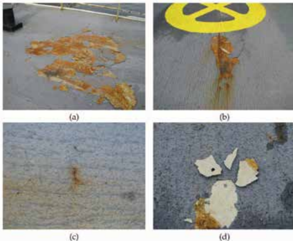
Figure 1 – Photographies du pont du gaillard du NCSM Glace Bay : (a, b) deux endroits montrant un large soulèvement du revêtement; (c) l'une des nombreuses petites fissures d'une longueur approximative de 1 cm que l'on trouve au hasard sur le pont; et (d) des morceaux de revêtement retirés aisément avec une petite spatule pour révéler une surface en parfait état en dessous.
