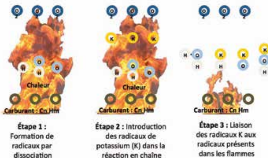
Figure 2 – Les particules de carbonate de potassium produites par un extincteur en aérosol éteignent un incendie de façon chimique en formant des molécules stables, comme de l'hydroxyde de potassium (KOH), qui interrompent l'accumulation d'hydroxyle (OH - ), d'oxygène (O + ) et d'hydrogène (H + ), des radicaux qui seraient autrement disponibles pour alimenter les réactions carburant-air dans les flammes.
