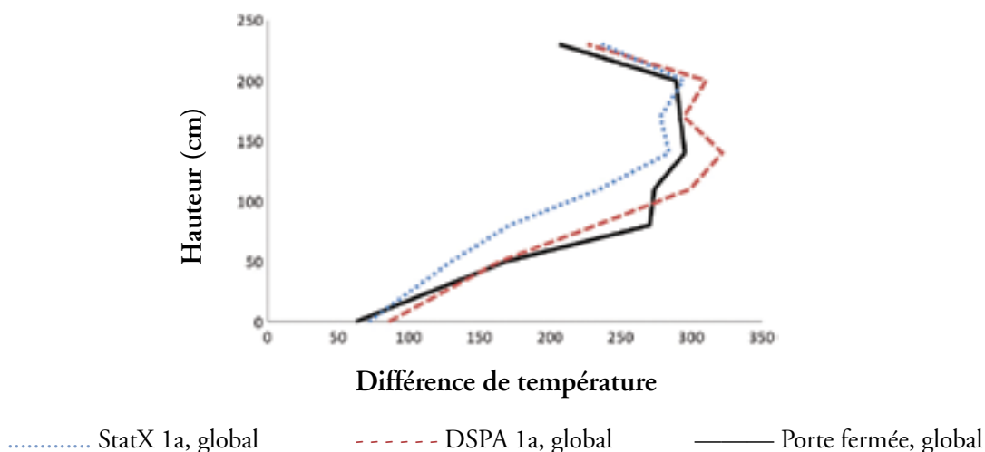
Figure 4 – Ce résumé de l'effet de refroidissement total du compartiment durant trois essais d'incendie ouvert alimenté au diesel montre que l'extinction à l'aide d'un aérosol seulement par les deux dispositifs d'essai était comparable à une extinction par privation d'oxygène seulement.
