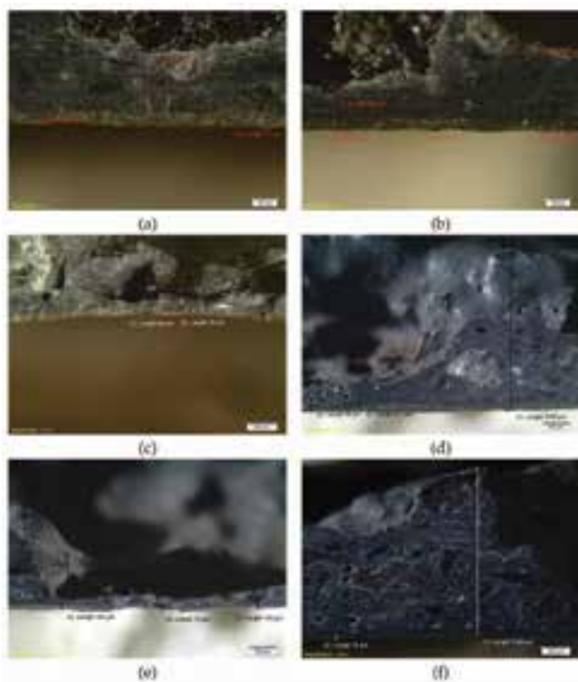
Figure 3 – Des images microscopiques de coupes transversales du revêtement. La couche argent-or plus mince correspond à l'apprêt, alors que la couche bleu-gris plus épaisse correspond à la couche de finition.
