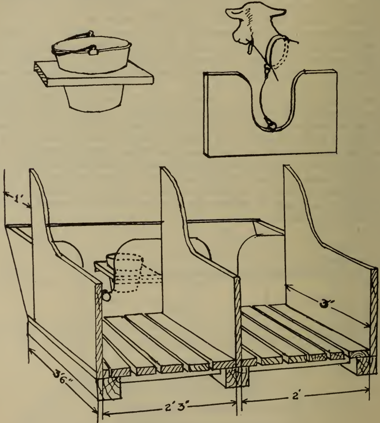
FIG. 9.—Plan d'une stalle pour les chèvres.
