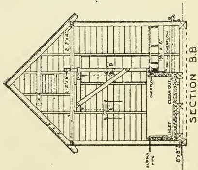
END ELEVATION
