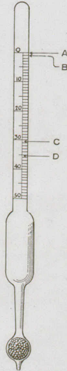
Fig. 29. SACCHAROMÈTRE
