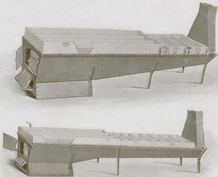
Fig. 16. MODÈLES D'ÉVAPORATEURS MODERNES Ils sont tous à fond plissé
