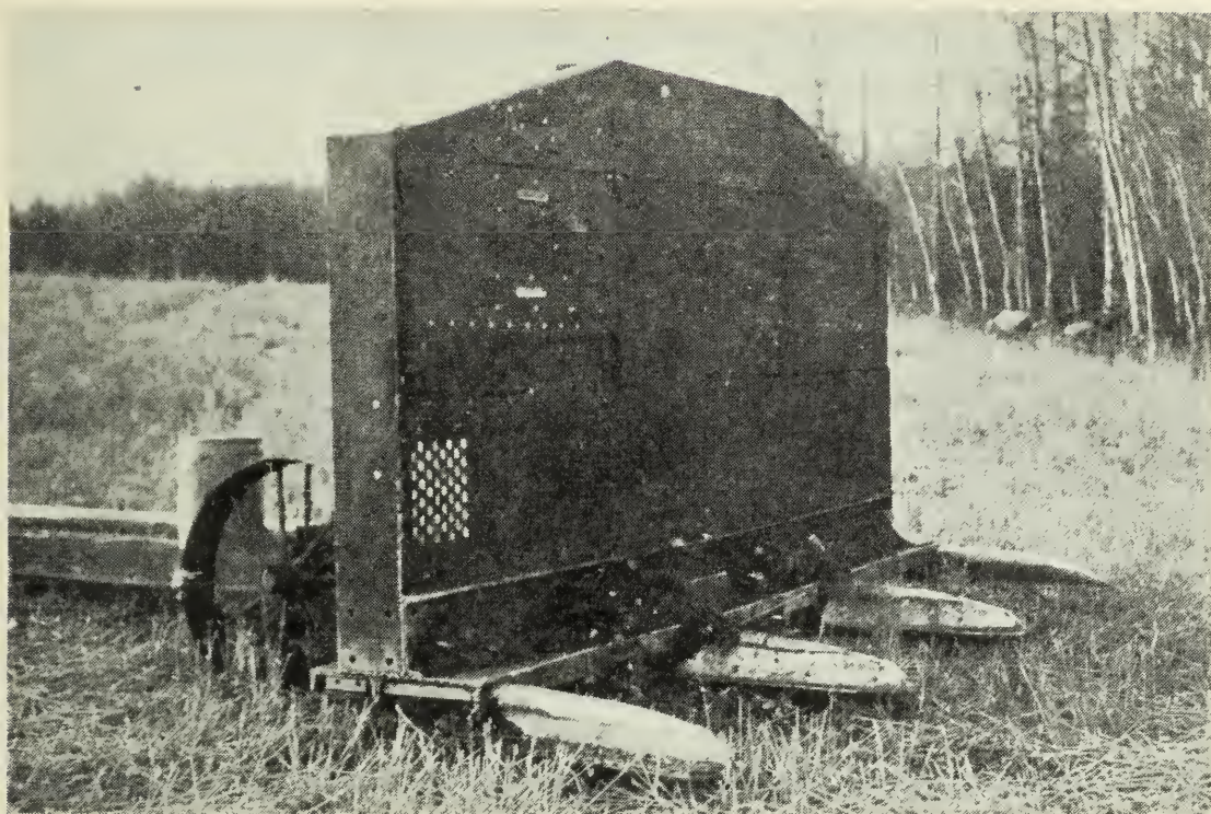
FIG. 5.—A piler.
