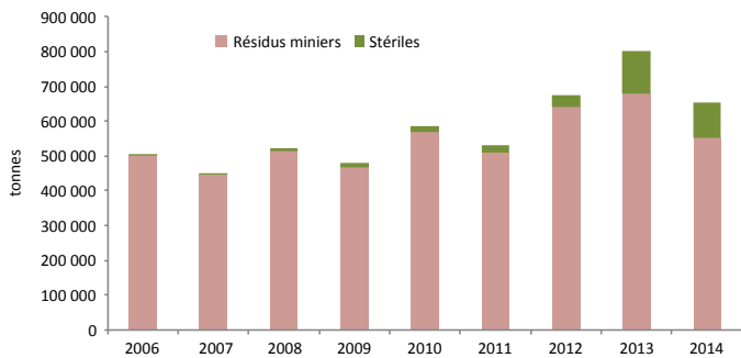
Figure 27 : Élimination de résidus miniers et de stériles, 2006-2014
