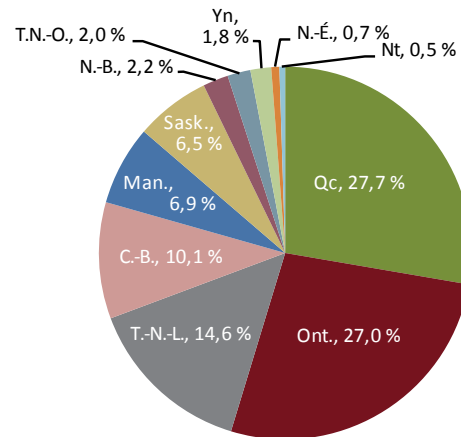
Figure 32 : Répartition régionale des tests de létalité aiguë pour la daphnie, 2004-2013
