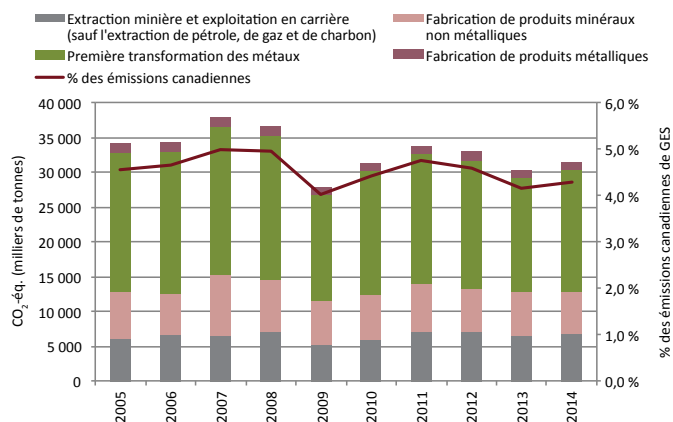
Figure 33 : Émissions de GES dans le secteur minier, 2005-2014
