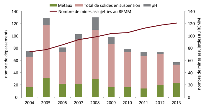
Figure 28 : Répartition des dépassements en vertu du REMM par substance, 2004-2013
