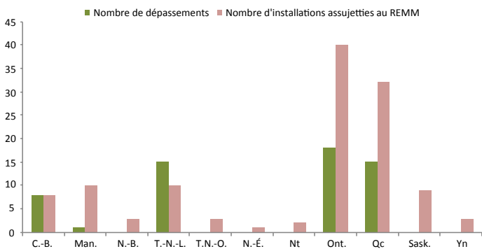
Figure 30 : Répartition régionale des installations et des dépassements, 2013
