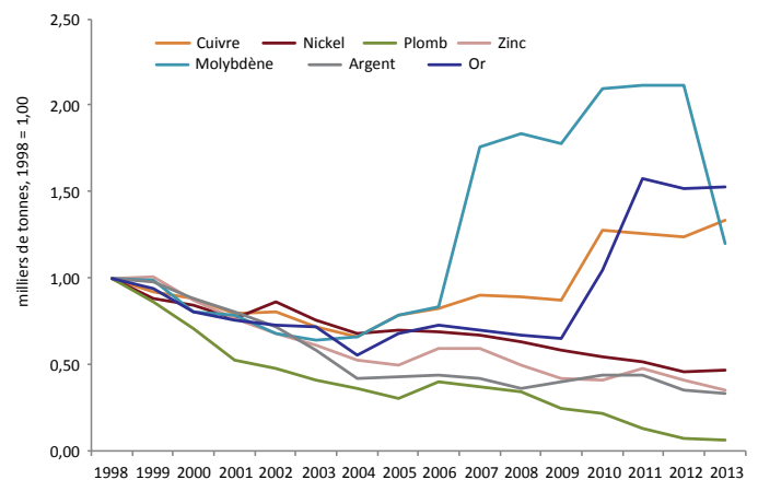
Figure 12 : Réserves canadiennes de métaux sélectionnés, 1998-2013
