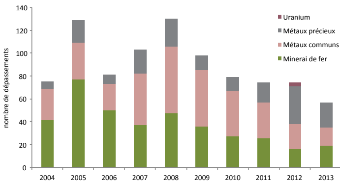
Figure 29 : Répartition des dépassements en vertu du REMM par sous-secteur, 2004-2013
