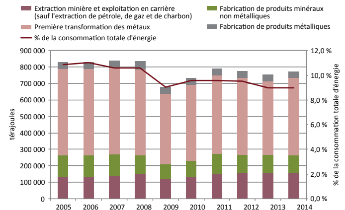
Figure 35 : Consommation d'énergie du secteur minier, 2005-2014
