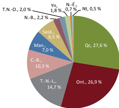
Figure 31 : Répartition régionale des tests de létalité aiguë pour la truite arc-en-ciel, 2004-2013
