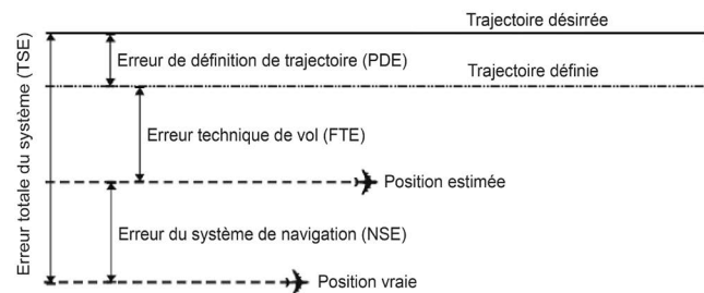
Figure 2.12 – Erreurs de navigation latérale
