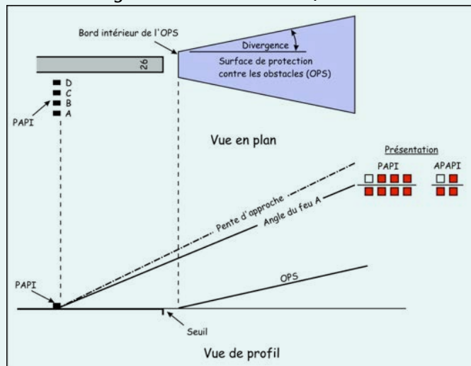
Figure 7.4 – OPS de PAPI/d'APAPI
