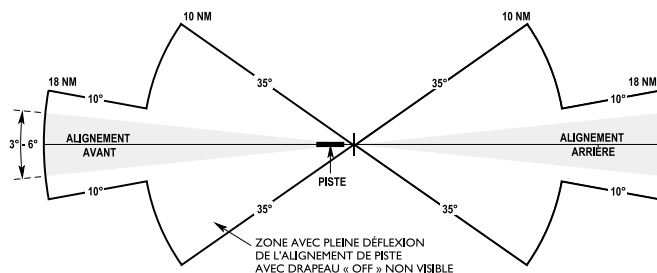
Figure 3.1 — Alignement avant et arrière du LOC
