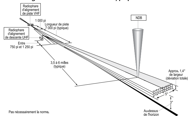
Figure 3.2 – Installation typique d'un ILS
