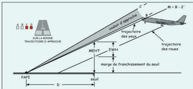
Figure 7.3 – PAPI – Trajectoire des yeux du pilote par rapport à la trajectoire des roues
