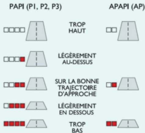
Figure 7.2 – Indications de PAPI et d'APAPI
