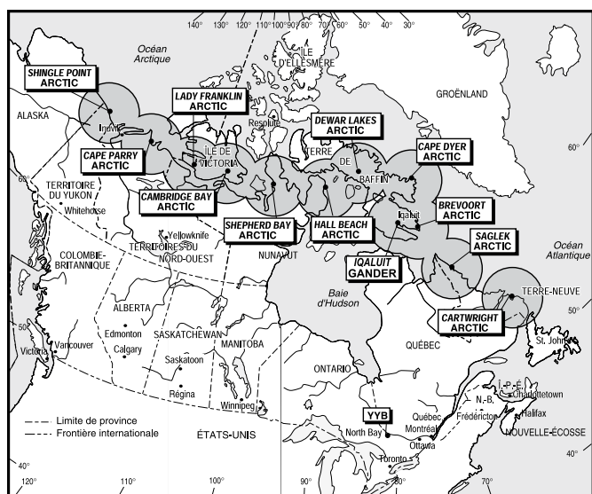
Figure 6.4 – Couverture VHF dans le nord du Canada – 30 000 pi
