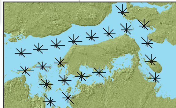
Figure 25 : Vents moyens en septembre, octobre et novembre, selon l'imagerie RADARSAT.
