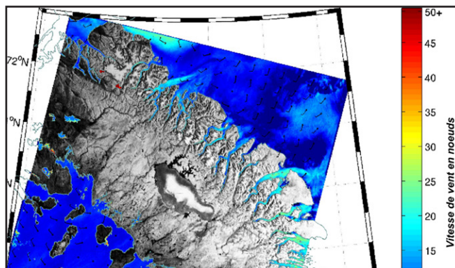
Figure 3 : Image RADARSAT du 15 septembre 2012 montrant des vents catabatiques modérés à forts.
