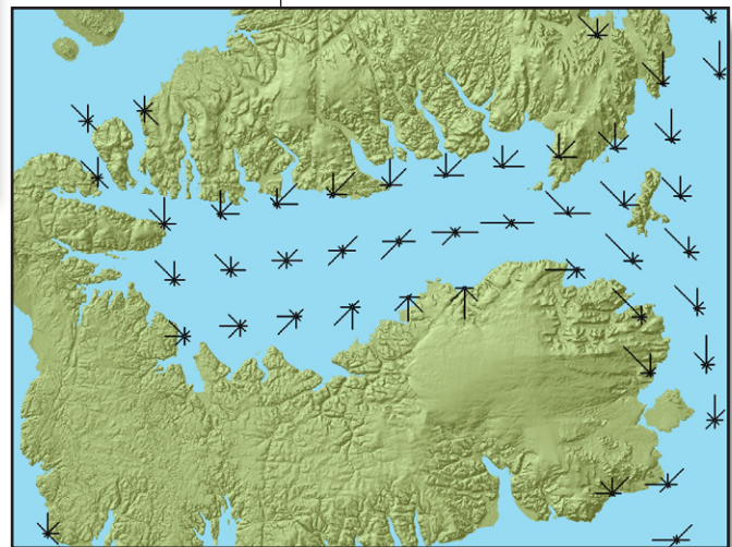
Figure 27 : Roses des vents d'après les données tirées de RADARSAT pour les mois de septembre, d'octobre et de novembre pour la région maritime de Jones.
