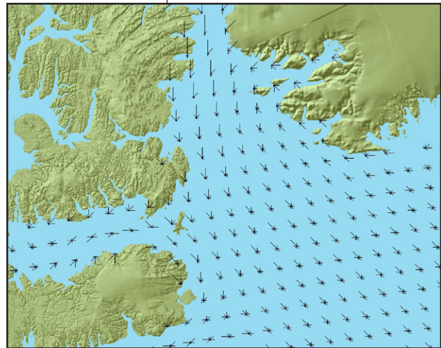
Figure 5 : Roses des vents d'après les données tirées de RADARSAT pour les mois de septembre, d'octobre et de novembre pour la région de Clarence.
