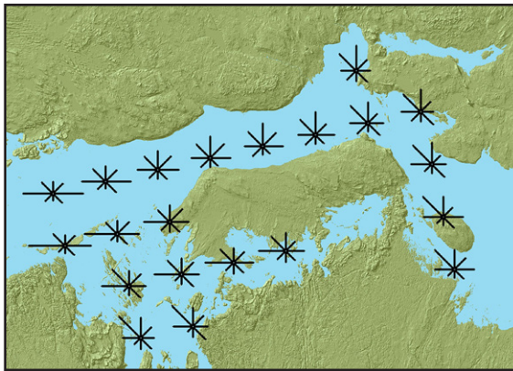
Figure 24 : Vents moyens en juin, juillet et août, selon l'imagerie RADARSAT.
