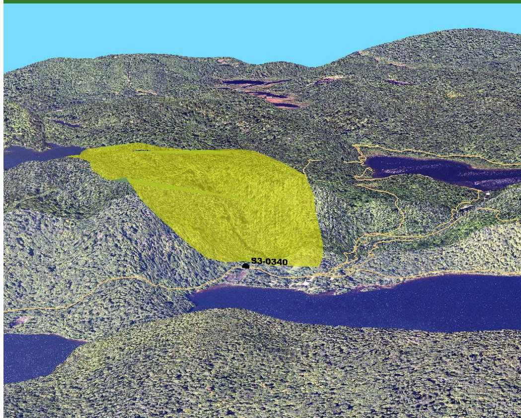
Figure 3 : Les débits d'eau de chaque ponceau sont fondés sur les caractéristiques du bassin hydrographique en amont des ponceaux en question. Le présent exemple montre la carte du bassin hydrographique qui se déverse dans le ponceau n° S3-0340.
