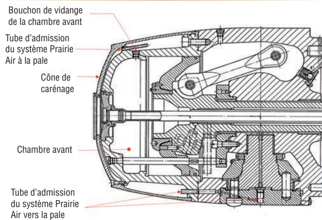
Schéma du moyeu d'hélice.
