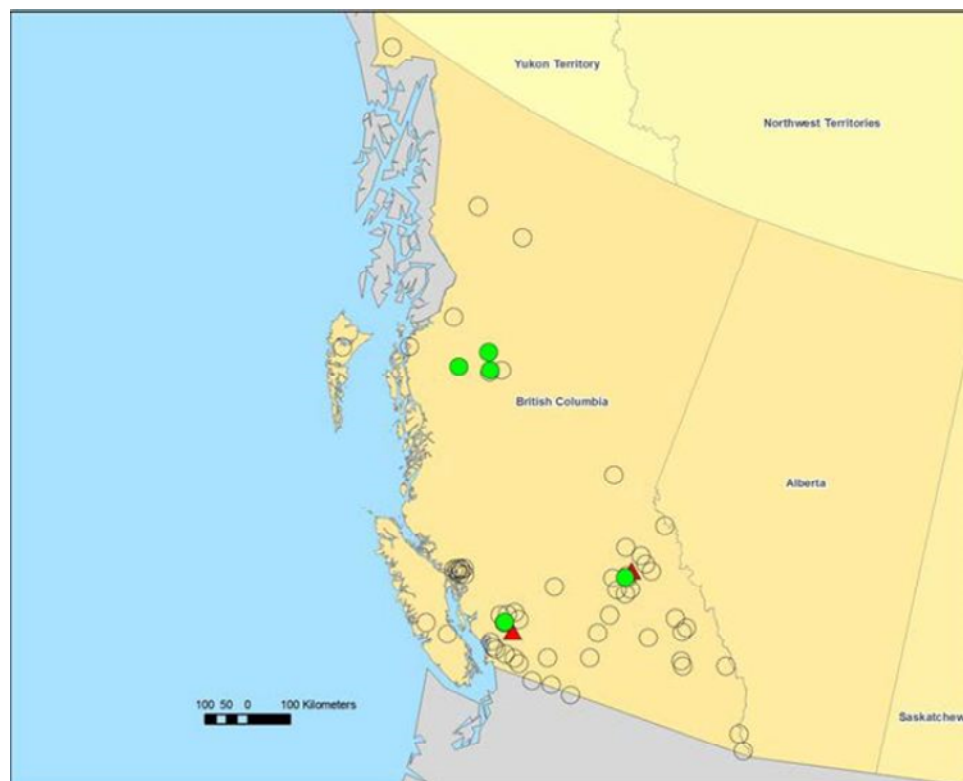
Figure 2. Répartition du peltigère éventail d'eau de l'Ouest en Colombie-Britannique. Les cercles verts indiquent l'emplacement des populations existantes; les cercles noirs indiquent les endroits où des recherches ont été effectuées, sans succès; les triangles rouges indiquent l'emplacement des occurrences historiques où l'espèce n'a pu être retrouvée lors des relevés effectués en 2011 et où elle est considérée comme étant disparue (COSEWIC, 2013).
