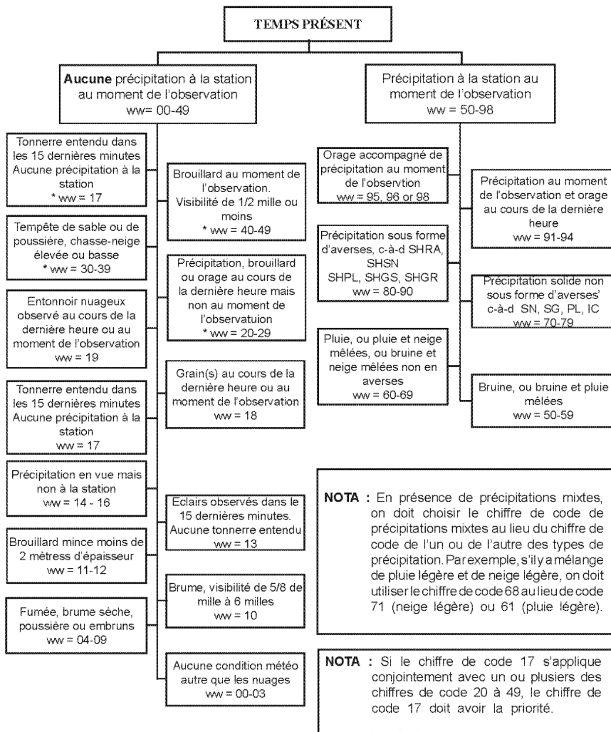
Figure 15—1 : Guide pour choisir les codes du temps présent
