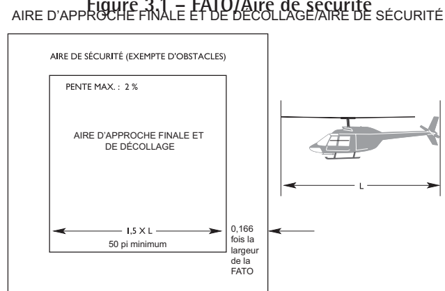
Figure 3.1 – FATO/Aire de sécurité
