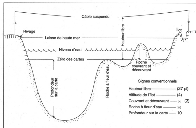
DIAGRAMME — ZÉRO DES CARTES, ALTITUDE, HAUTEUR LIBRE
