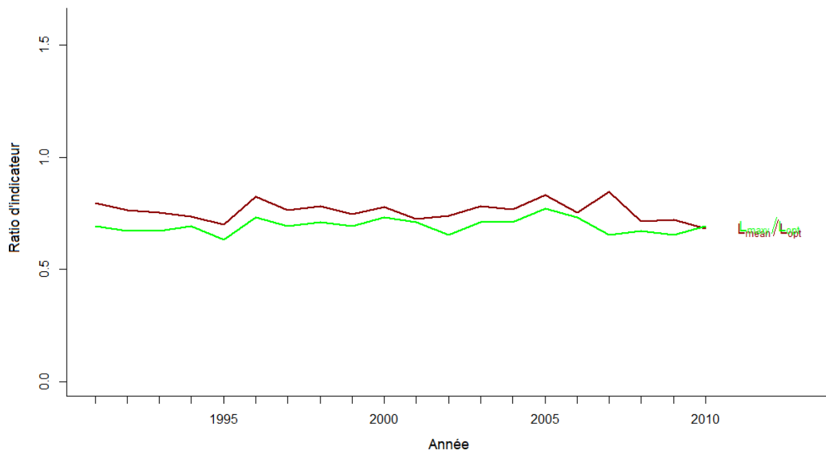
Figure A.3. Série temporelle des indicateurs du rendement optimal d'ICES (graphique du haut) et de leur ratio par rapport à des points de référence (graphique du bas) basée sur la longueur dans les prises commerciales de la plie canadienne dans la zone de pêche 4T de l'OPANO de 1991 à 2010.
