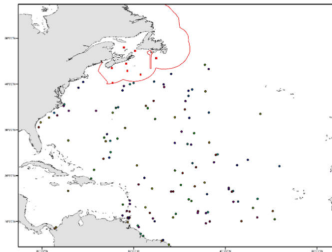
Figure 2. L'emplacement des dernières transmissions d'étiquettes émettrices de 133 tortues luths a fait l'objet d'un suivi dans les eaux canadiennes.
