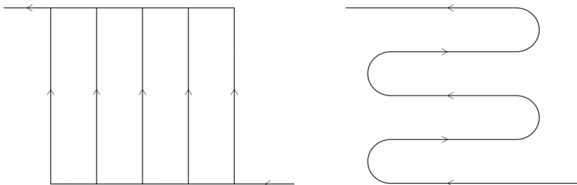
Configuration en collecteur avec 5 longueurs parallèles
