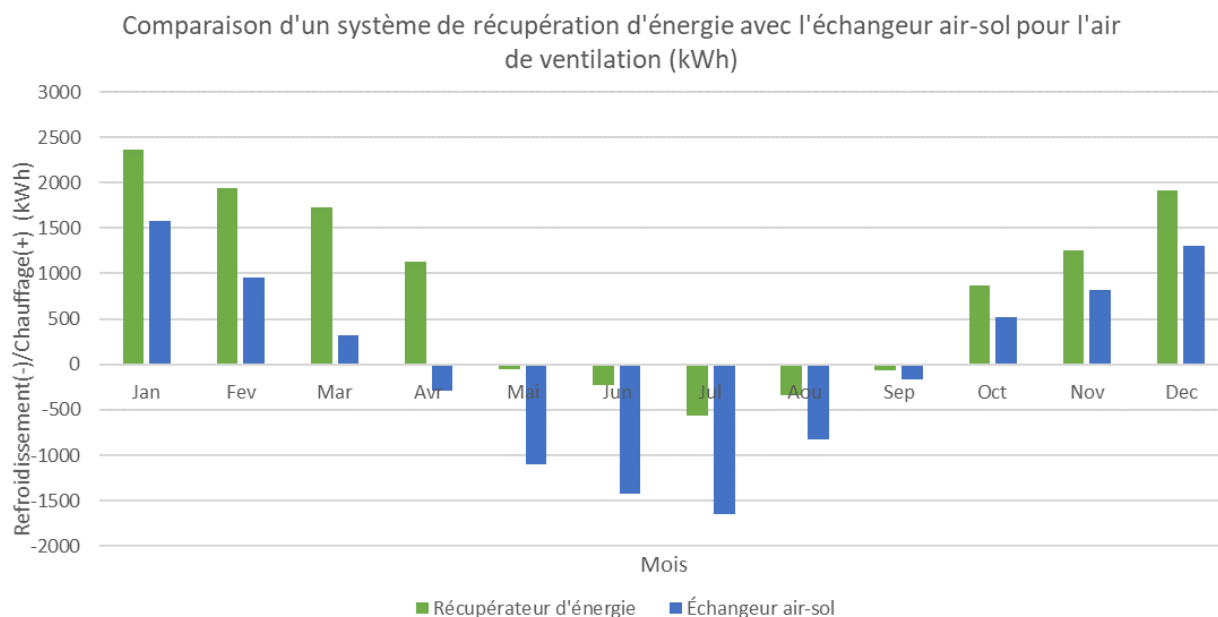
Figure 12 : Comparaison entre les systèmes d'échangeurs thermiques terre-airs et les systèmes de récupération de l'énergie
