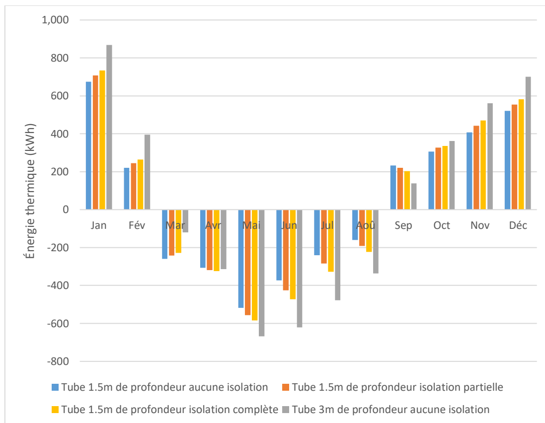
Figure 3 : Effet de l'installation d'un isolant au-dessus du tube souterrain
