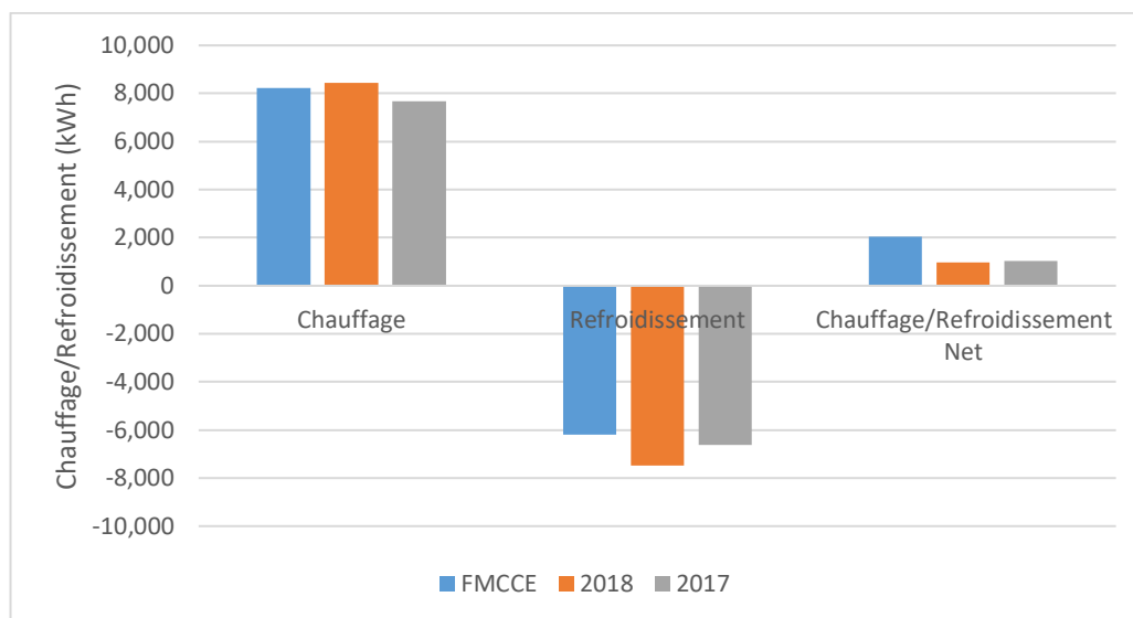
Figure 18 : Production de chauffage, refroidissement et bilan net annuel
