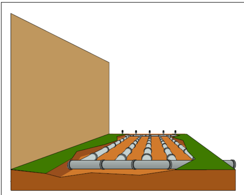
Figure 8d : Plusieurs tubes distributeurs connectés au collecteur
