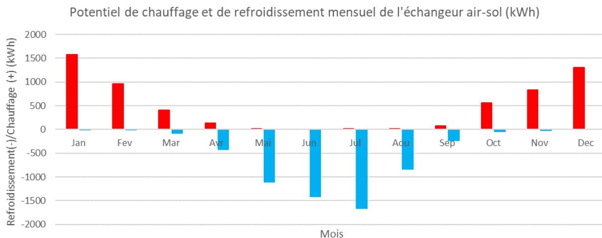
Figure 11 : Potentiel mensuel total de chauffage et de refroidissement
