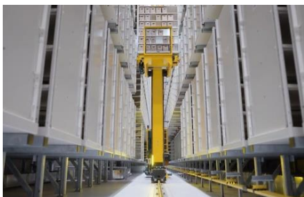
Le système de rayonnage et de récupération automatisé
