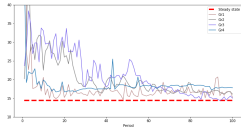
(d) \lambda = 3.9
