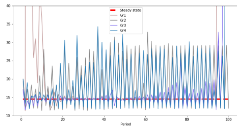
(d) \lambda = 3.83
