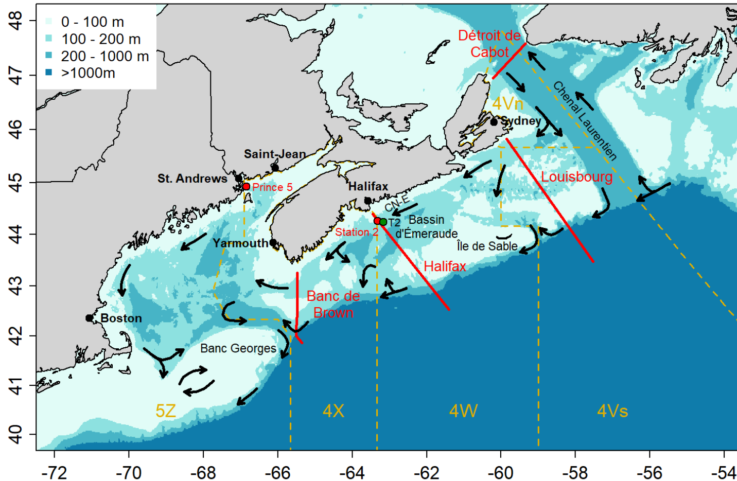
Figure 1. Carte du plateau néo-écossais et du golfe du Maine montrant les stations hydrographiques (cercles rouges), les sections standards (lignes rouges), le mouillage du courantmètre (vert) ainsi que les caractéristiques topographiques. Le Courant de la Nouvelle-Écosse (NSC) est indiqué. Les lignes pointillées indiquent les limites des divisions de l'Organisation des pêches de l'Atlantique Nord-Ouest.
