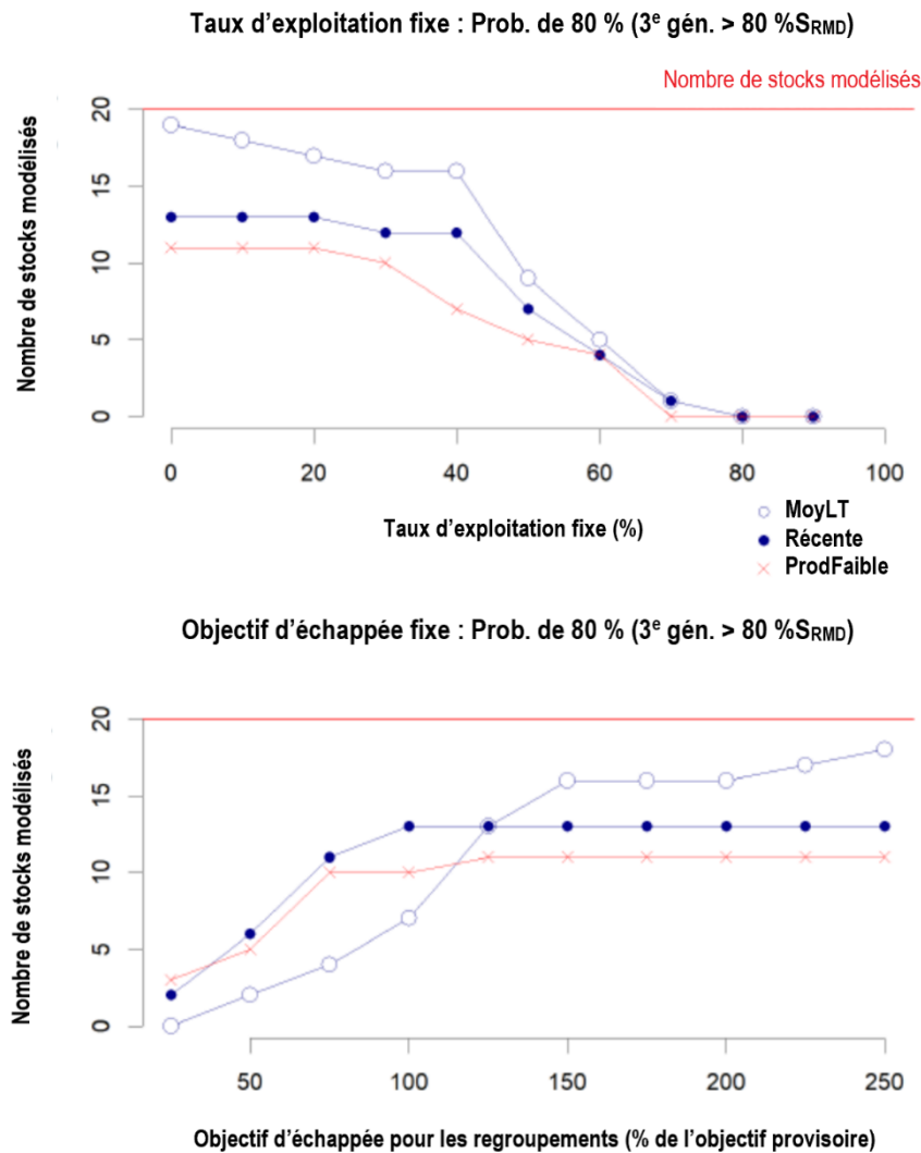
Figure 5. Exemples de simulations prospectives simples – toutes les variantes. Les graphiques montrent le nombre de stocks ayant une probabilité d'au moins 80 % de respecter un point de référence fixé à 80 % de la médiane de S_{RMD} pour le scénario de productivité moyenne à long terme. Les résultats sont présentés dans trois scénarios de productivité pour 10 niveaux de taux d'exploitation fixe pour les regroupements et 10 niveaux d'échappée fixe pour les regroupements (exprimés en % de l'objectif d'échappée provisoire pour les deux groupes modélisés, rivière Nass et stock sauvage de la rivière Skeena).
