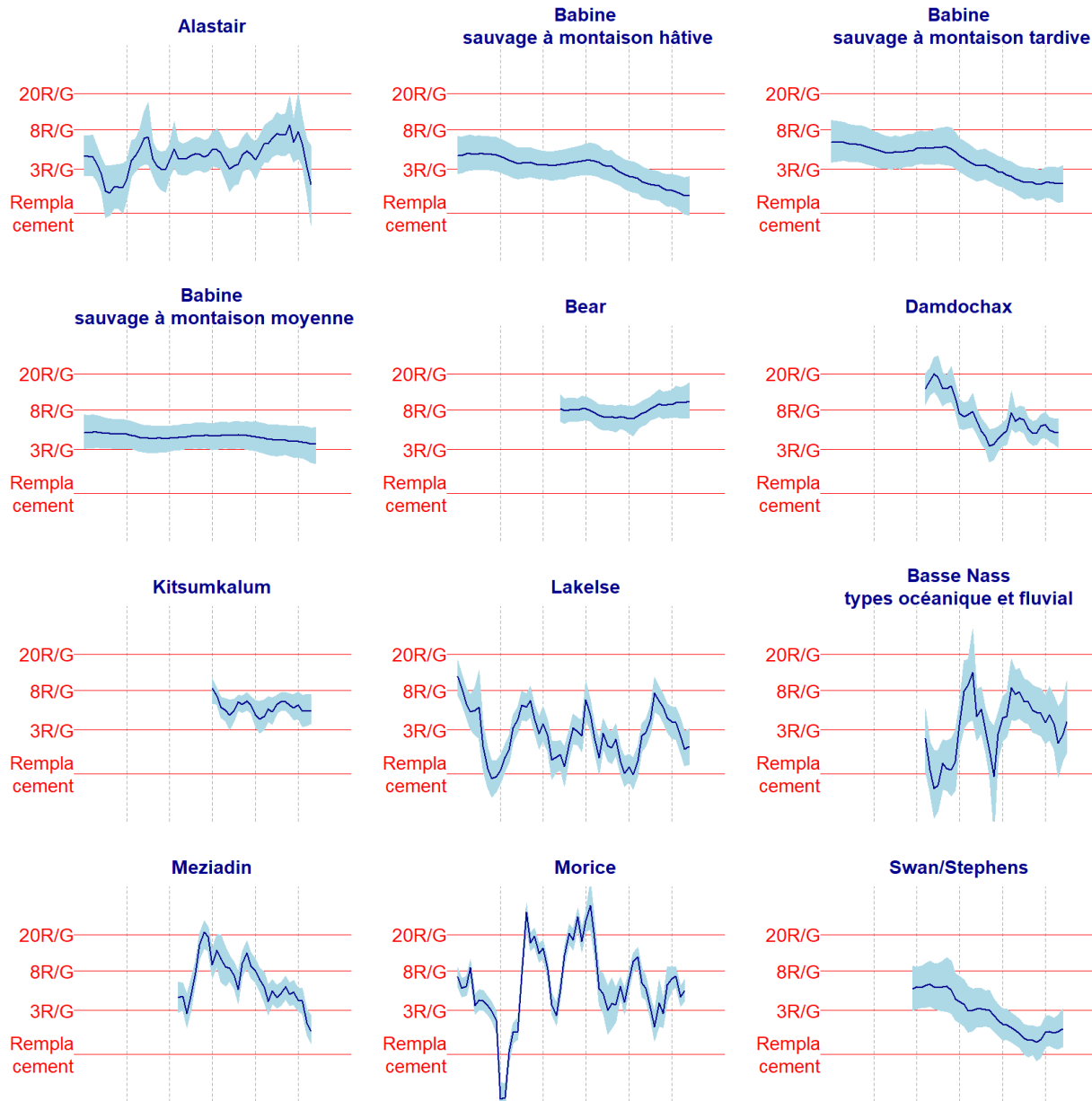
Figure 3. Tendence de la productivité variable dans le temps pour 12 stocks pour lesquels on dispose d'une série chronologique complète. Chaque graphique montre la médiane et les limites de 80 % des distributions a posteriori de \ln(\alpha) , par année, pour le modèle géniteurs-recrues ajusté avec un \alpha variable dans le temps. Les lignes de référence indiquent la productivité intrinsèque correspondante en matière de recrues par géniteur (R/G) à une très faible abondance de géniteurs (techniquement, à 0 géniteur).
