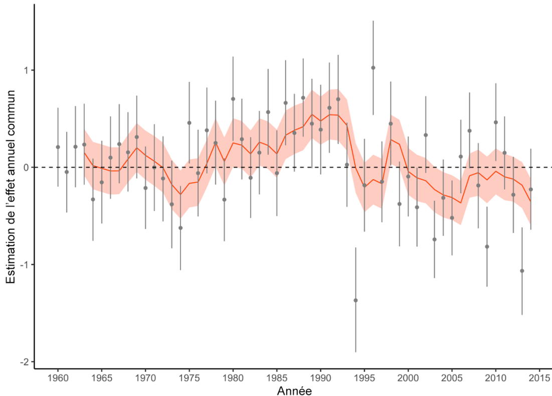
Figure 4. Estimation de l'effet annuel commun aux 18 stocks de la rivière Skeena avec une moyenne mobile sur quatre ans. Les points indiquent la moyenne avec les barres d'erreur représentant les intervalles crédibles à 95 %, tandis que la ligne et l'ombrage dénotent la moyenne et les intervalles crédibles à 95 % pour la moyenne mobile.
